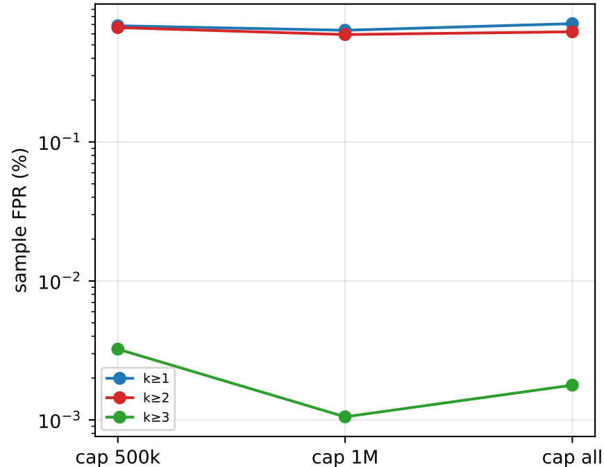
Fusion FPR vs benign cap
