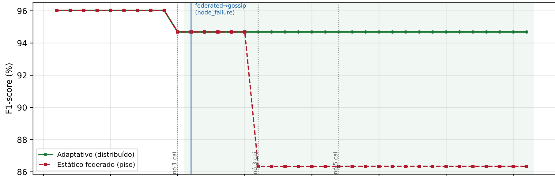
ERENO v2 — 14 nós, k \geq 2 : adaptativo (FL->GL) vs estático sob perda de sensores
