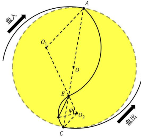
图 18 情况三判断角示意图
