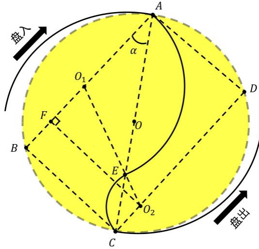
图 16 调头路径示意图
