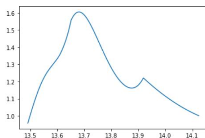
图 29 龙头进入盘出螺线的过程中，第三节龙身前把手的速度
