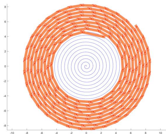
图 14 最小螺距下最接近碰撞时刻示意图
