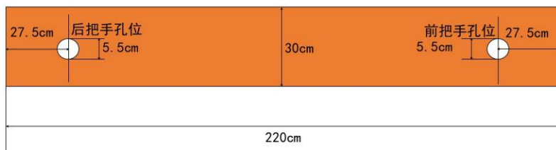
图 2 龙身、龙尾俯视数据图
