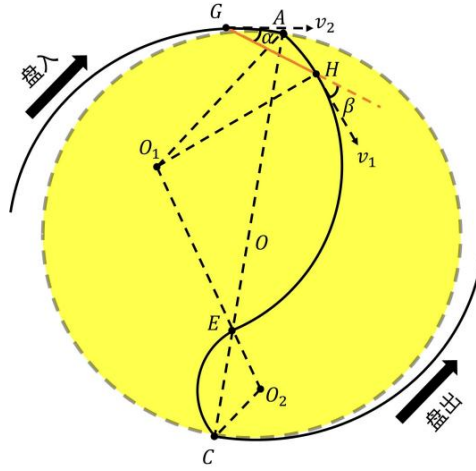
图 25 速度迭代示意图
