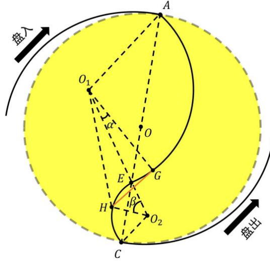
图 22 情况四示意图
