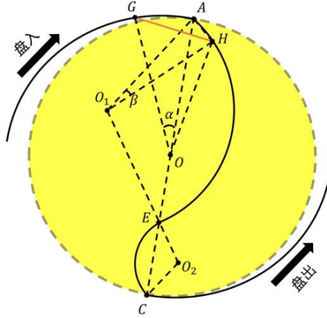
图 20 情况二示意图
