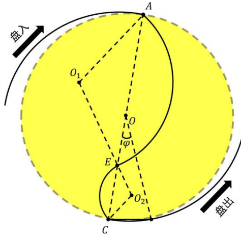
图 19 情况四判断角示意图
