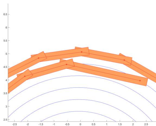
图 15 最小螺距下最接近碰撞时刻示意图（放大）
