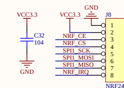
NRF2401无线通信接口
