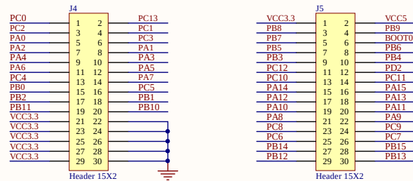
通用IO接口
