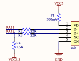
USB 5V供电
