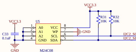
EEPROM-存储数据
