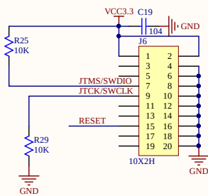
JTAG调试接口
