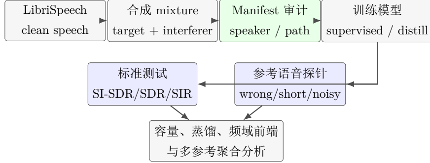
图 3 数据构造、训练与评估流程。数据审计和参考语音探针用于保证模型确实学习目标说话人条件。
