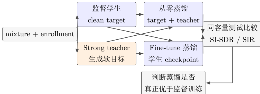
图 4 知识蒸馏实验设计。本文将同架构监督学生、从零蒸馏和 fine-tune 蒸馏放在同一测试集上比较。
