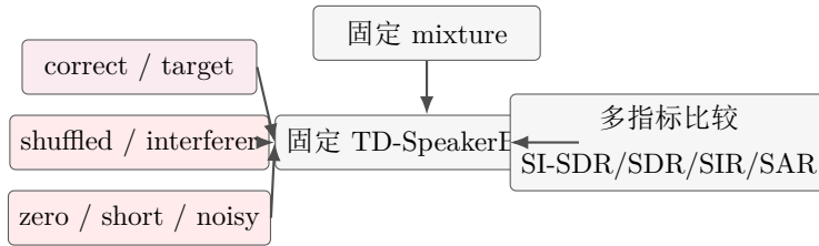
图 5 Enrollment sanity check 设计。固定 mixture 和模型，仅替换参考语音以验证目标身份条件是否生效。
