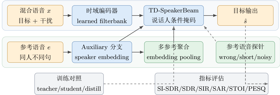
图 2 目标说话人提取系统结构。实线为分离主路径，虚线为训练、诊断和多参考聚合环节。
