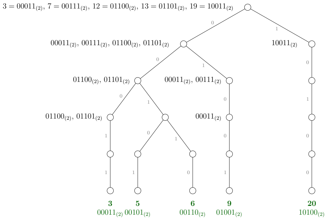
Figura 39.1: Trie-ul construit pentru exemplul 2 din enunț, în care dorim să obținem al k = 10 -lea cel mai mic xor. În rădăcină obținem 4 \cdot 4 + 1 \cdot 1 = 17 perechi cu xor-ul 0, deci primul bit al răspunsului este 0. Pe nivelul 1 (corespunzător celui de-al doilea bit din stînga) obținem 2 \cdot 3 + 2 \cdot 1 + 1 \cdot 1 = 9 perechi cu xor-ul 0, deci al doilea bit al rezultatului este 1.
