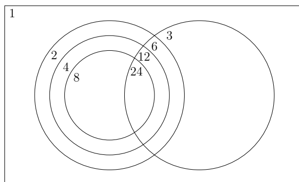
Figura 21.2: O colecție redundantă de mulțimi.
