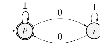
Figura 35.1: Un exemplu de automat finit determinist.
