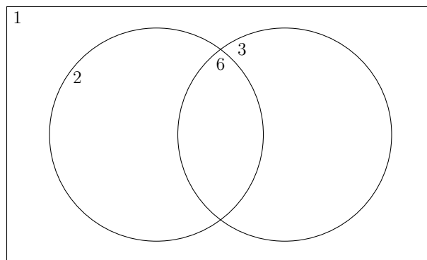
Figura 21.1: Mulțimile pentru coprimalitatea cu 24.
