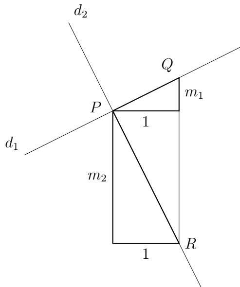
Figura 25.1: Dreptele d_1 și d_2 au respectiv pantele m_1 și m_2 .
