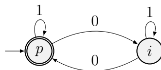
Figura 35.1: Un exemplu de automat finit determinist.
