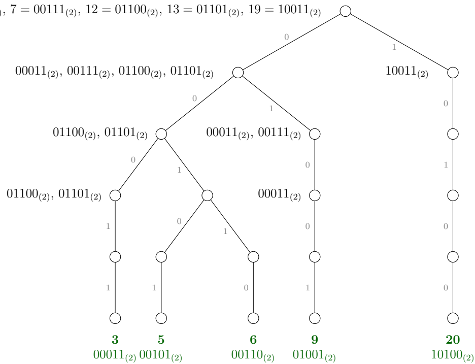
Figura 39.1: Trie-ul construit pentru exemplul 2 din enunț, în care dorim să obținem al k = 10 -lea cel mai mic xor. În rădăcină obținem 4 \cdot 4 + 1 \cdot 1 = 17 perechi cu xor-ul 0, deci primul bit al răspunsului este 0. Pe nivelul 1 (corespunzător celui de-al doilea bit din stînga) obținem 2 \cdot 3 + 2 \cdot 1 + 1 \cdot 1 = 9 perechi cu xor-ul 0, deci al doilea bit al rezultatului este 1.
