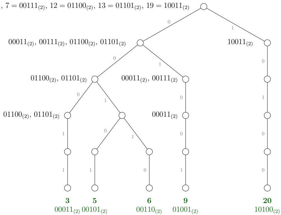
Figura 41.1: Trie-ul construit pentru exemplul 2 din enunț, în care dorim să obținem al k = 10 -lea cel mai mic xor. În rădăcină obținem 4 \cdot 4 + 1 \cdot 1 = 17 perechi cu xor-ul 0, deci primul bit al răspunsului este 0. Pe nivelul 1 (corespunzător celui de-al doilea bit din stînga) obținem 2 \cdot 3 + 2 \cdot 1 + 1 \cdot 1 = 9 perechi cu xor-ul 0, deci al doilea bit al rezultatului este 1.
