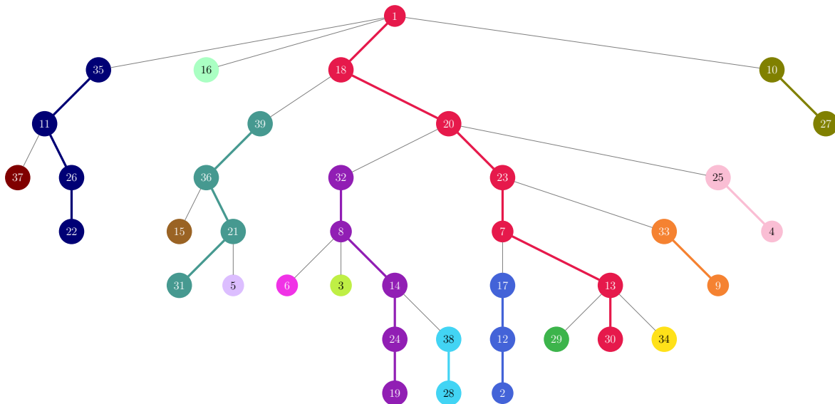
Figura 20.1: Un arbore în care muchia grea a fiecărui nod este îngroșată și colorată. Fiecare culoare indică un lanț de muchii grele consecutive.
