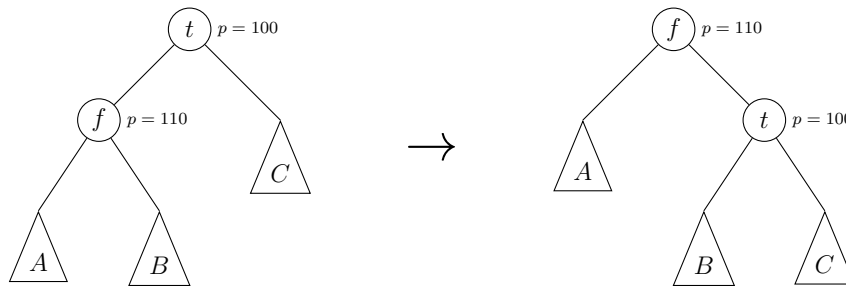
Figura 12.2: Rotația spre dreapta a unui subarboare. Rotația spre stînga funcționează simetric.
