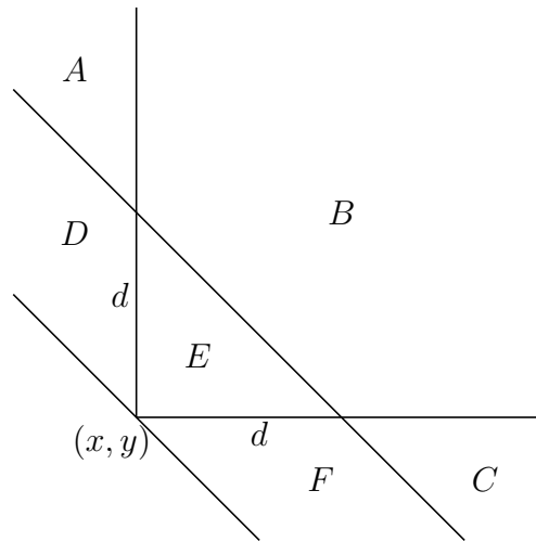
Figura 28.4: Poziția liniei de baleiere la două evenimente cauzate de interogarea triunghiulară E : baza și vârful triunghiului.
