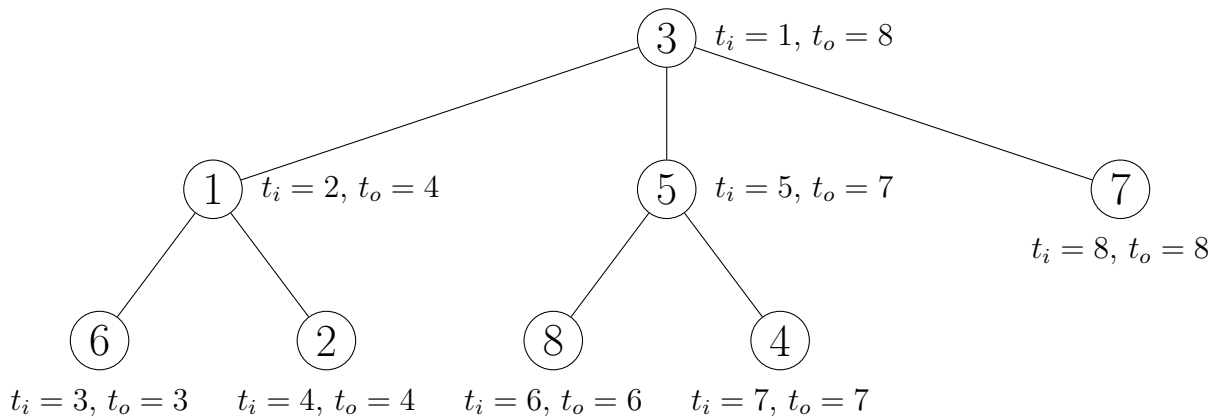
Figura 16.2: Timpii de intrare și de ieșire din noduri, varianta 2.
