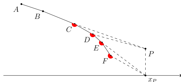
Figura 28.3: Punctul (x_P, 0) șterge vrăjitorii F și E din stivă. Apoi, punctul P șterge vrăjitorii D și C din stivă. Unghiurile marcate cu roșu sînt reflexe.
