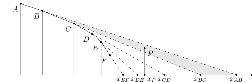
Figura 28.2: Mentorul vrăjitorului P este D deoarece x_P se află în triunghiul lui D . Mai mult, punctul P se află în triunghiul lui B , deci vrăjitorii C - F nu vor mai fi mentori niciodată.
