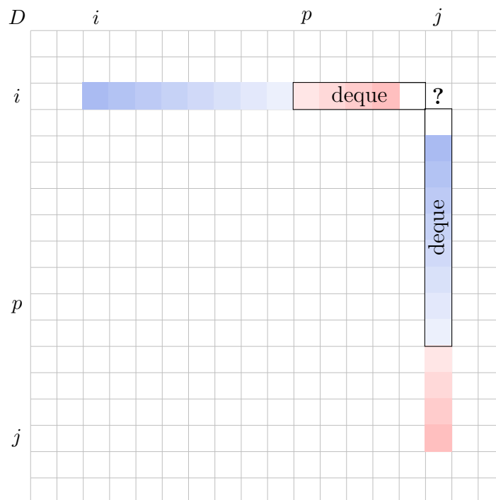
Figura 42.1: Matricea D și zonele de interes pentru calculul lui D_{i,j} .
