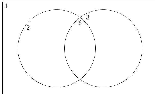
Figura 22.1: Mulțimile pentru coprimalitatea cu 24.
