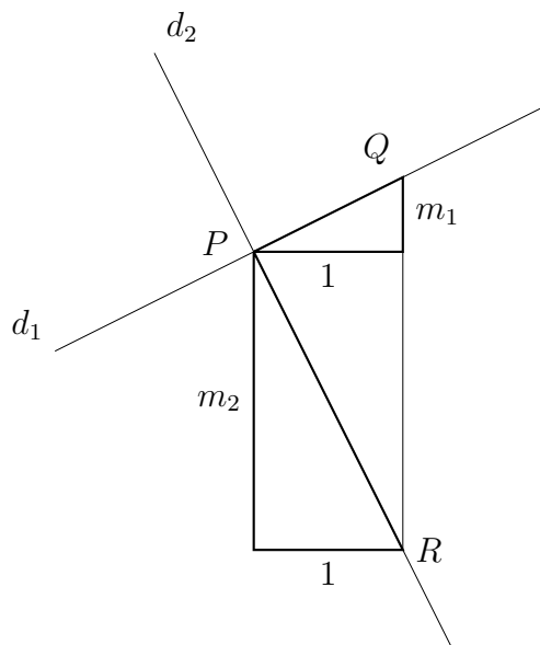
Figura 27.1: Dreptele d_1 și d_2 au respectiv pantele m_1 și m_2 .
