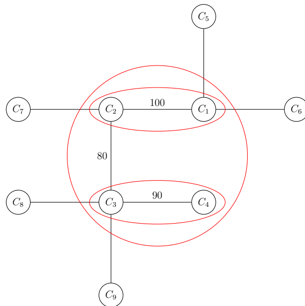
Figura 30.1: Unificarea componentelor biconexe prin punți.
