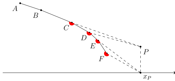
Figura 24.3: Punctul (x_P, 0) șterge vrăjitorii F și E din stivă. Apoi, punctul P șterge vrăjitorii D și C din stivă. Unghiurile marcate cu roșu sînt reflexe.
