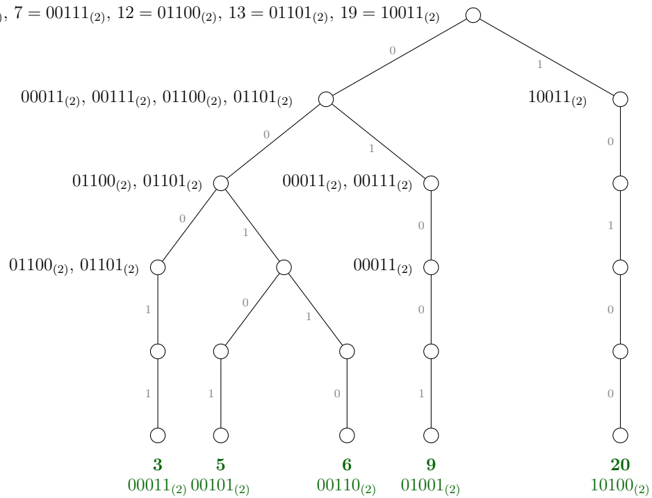
Figura 37.1: Trie-ul construit pentru exemplul 2 din enunț, în care dorim să obținem al k = 10 -lea cel mai mic xor. În rădăcină obținem 4 \cdot 4 + 1 \cdot 1 = 17 perechi cu xor-ul 0, deci primul bit al răspunsului este 0. Pe nivelul 1 (corespunzător celui de-al doilea bit din stînga) obținem 2 \cdot 3 + 2 \cdot 1 + 1 \cdot 1 = 9 perechi cu xor-ul 0, deci al doilea bit al rezultatului este 1.
