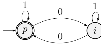
Figura 30.1: Un exemplu de automat finit determinist.
