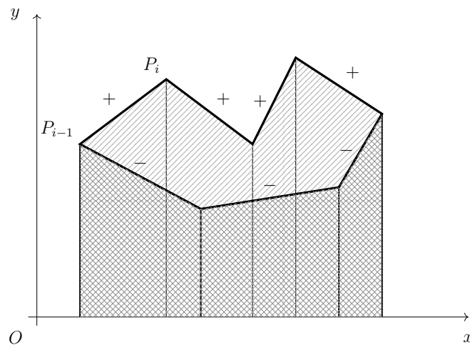
Figura 20.2: Aria heptagonului cu contur gros se obține prin însumarea ariilor cu semn ale celor 7 trapeze.
