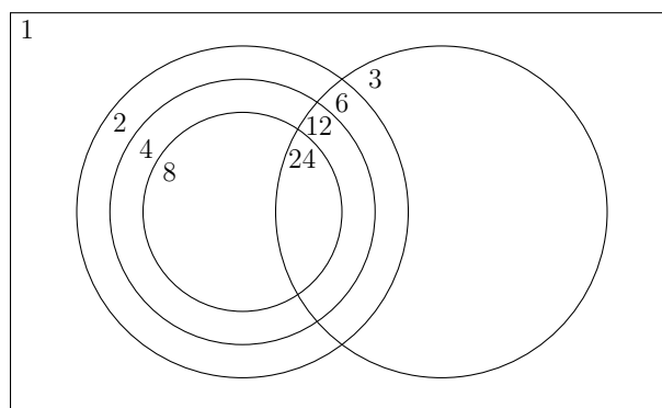
Figura 23.2: O colecție redundantă de mulțimi.
