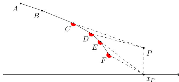
Figura 29.3: Punctul (x_P, 0) șterge vrăjitorii F și E din stivă. Apoi, punctul P șterge vrăjitorii D și C din stivă. Unghiurile marcate cu roșu sînt reflexe.
