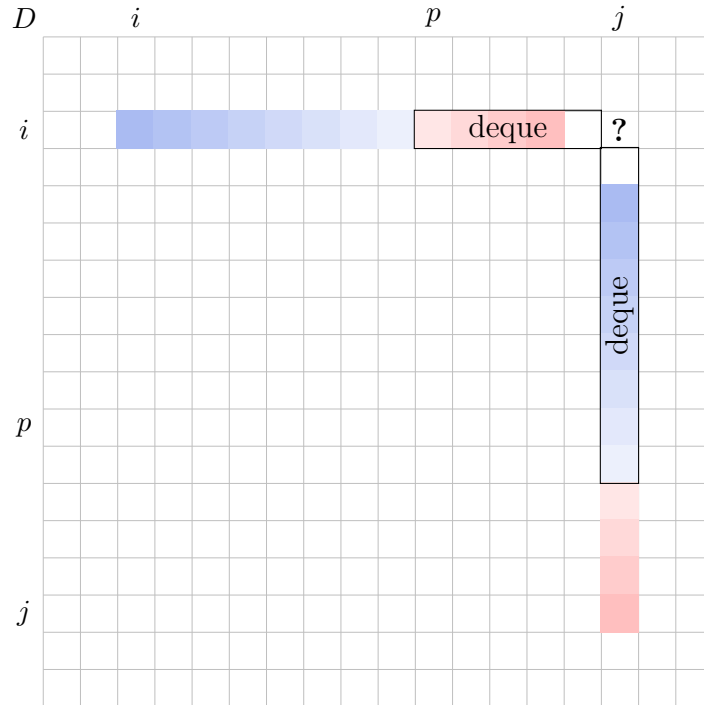
Figura 43.1: Matricea D și zonele de interes pentru calculul lui D_{i,j} .
