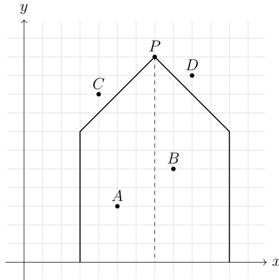
Figura 7.1: Zona de acoperire a festivalului P pentru d = 4 . Punctul P poate fi vizitat după punctele A sau B , dar nu și după C sau D .
