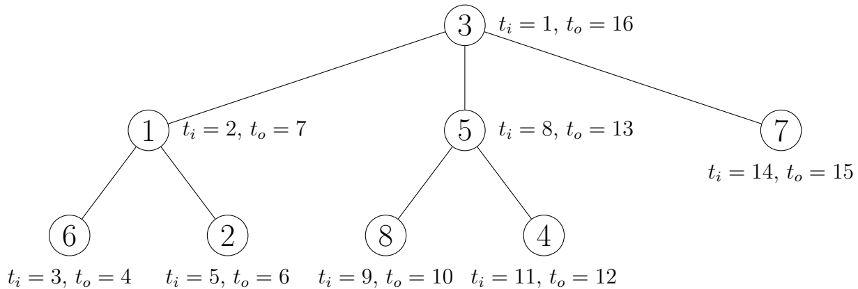
Figura 17.1: Timpii de intrare și de ieșire din noduri, varianta 1.
