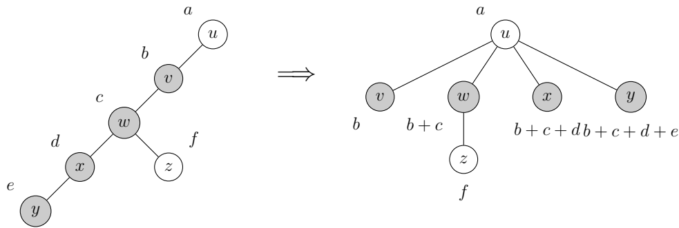
Figura 31.2: Compresia căii u - y . Când legăm nodurile w , x și y (și v ) direct de rădăcina u , le recalculăm costurile astfel încât sumele pe căi să rămână neschimbate, respectiv a + b (pe calea de la u la v ), a + b + c (pe carea de la u la w ) etc. Nodurile din afara căii nu necesită modificări. Costul pe calea de la u la z rămâne a + b + c + f .
