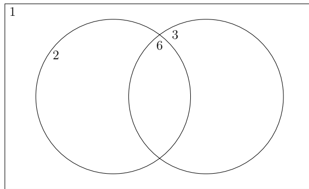
Figura 23.1: Mulțimile pentru coprimalitatea cu 24.
