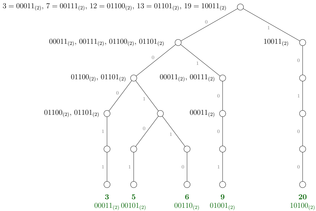
Figura 36.1: Trie-ul construit pentru exemplul 2 din enunț, în care dorim să obținem al k = 10 -lea cel mai mic xor. În rădăcină obținem 4 \cdot 4 + 1 \cdot 1 = 17 perechi cu xor-ul 0, deci primul bit al răspunsului este 0. Pe nivelul 1 (corespunzător celui de-al doilea bit din stînga) obținem 2 \cdot 3 + 2 \cdot 1 + 1 \cdot 1 = 9 perechi cu xor-ul 0, deci al doilea bit al rezultatului este 1.
