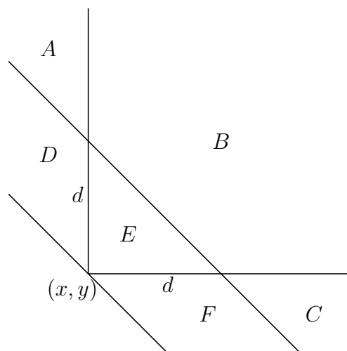
Figura 22.4: Poziția liniei de baleiere la două evenimente cauzate de interogarea triunghiulară E : baza și vârful triunghiului.
