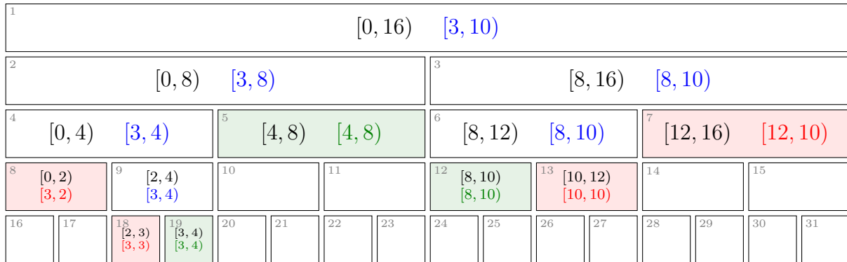
Figura 3.2: Arborele de apeluri în funcția de actualizare recursivă pe intervalul [3, 10) .
