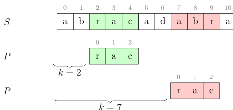
Figura 30.1: Pentru șablonul P = \text{rac} și șirul S = \text{abracadabra} , k = 2 este o deplasare validă, iar k = 7 este o deplasare invalidă.
