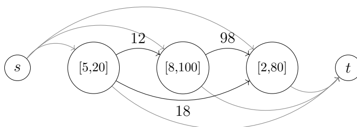
Figura 29.1: O încercare de graf pentru problema Lifts. Toate capacitățile sînt 1 și toate costurile sînt 0, cu excepția celor figureate pe muchii.
