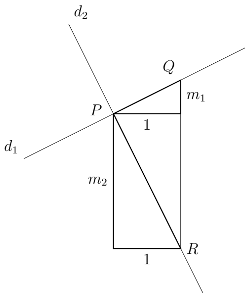
Figura 21.1: Dreptele d_1 și d_2 au respectiv pantele m_1 și m_2 .
