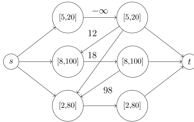
Figura 29.2: O nouă încercare de graf pentru problema Lifts.
