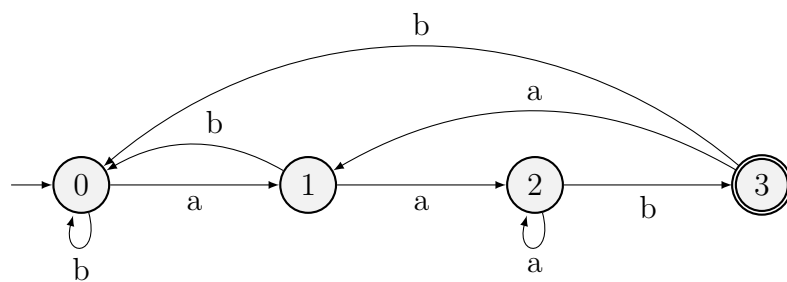
Figura 31.6: Un automat care recunoaște aparițiile subșirului aab .
