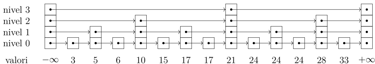
Figura 8.1: O listă pe niveluri, utilă pentru date statice.
