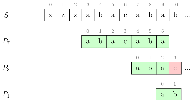
Figura 31.8: La poziția 10, nu putem extinde prefixul P_3 cu caracterul b , ci numai prefixul P_1 .
