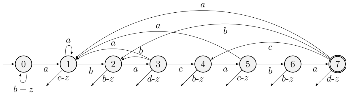
Figura 31.7: Un automat care recunoaște aparițiile subșirului abacaba . Săgețile de sub fiecare nod duc înapoi în starea 0.
