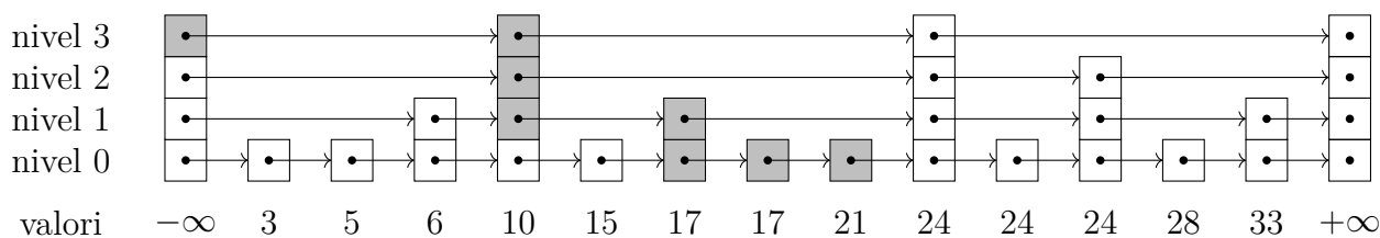
Figura 8.2: O listă pe niveluri probabilistică. Pointerii colorați cu gri sînt cei consultați pe parcursul căutării valorii 21.
