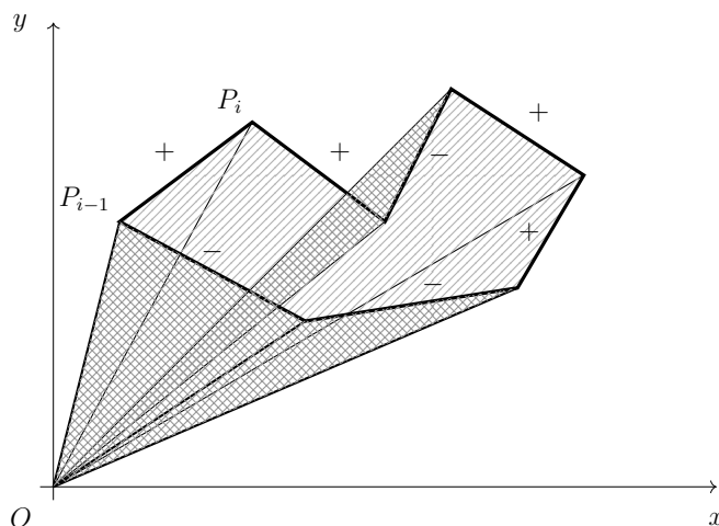
Figura 21.3: Aria heptagonului cu contur gros se obține prin însumarea ariilor cu semn ale celor 7 triunghiuri.
