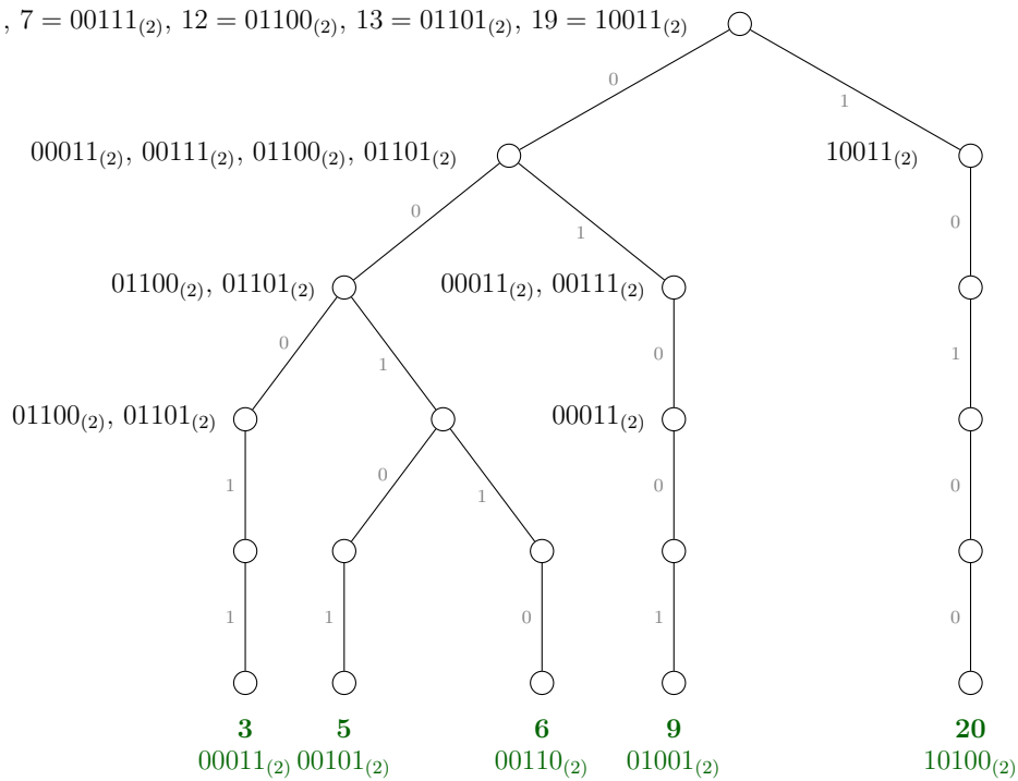
Figura 35.1: Trie-ul construit pentru exemplul 2 din enunț, în care dorim să obținem al k = 10 -lea cel mai mic xor. În rădăcină obținem 4 \cdot 4 + 1 \cdot 1 = 17 perechi cu xor-ul 0, deci primul bit al răspunsului este 0. Pe nivelul 1 (corespunzător celui de-al doilea bit din stînga) obținem 2 \cdot 3 + 2 \cdot 1 + 1 \cdot 1 = 9 perechi cu xor-ul 0, deci al doilea bit al rezultatului este 1.
