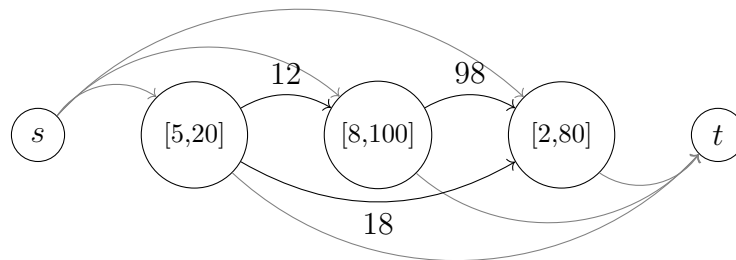
Figura 34.1: O încercare de graf pentru problema Lifts. Toate capacitățile sînt 1 și toate costurile sînt 0, cu excepția celor figureate pe muchii.
