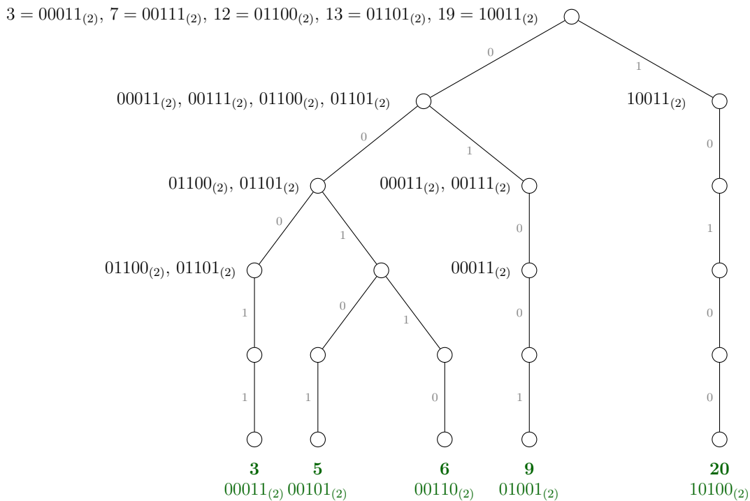
Figura 40.1: Trie-ul construit pentru exemplul 2 din enunț, în care dorim să obținem al k = 10 -lea cel mai mic xor. În rădăcină obținem 4 \cdot 4 + 1 \cdot 1 = 17 perechi cu xor-ul 0, deci primul bit al răspunsului este 0. Pe nivelul 1 (corespunzător celui de-al doilea bit din stînga) obținem 2 \cdot 3 + 2 \cdot 1 + 1 \cdot 1 = 9 perechi cu xor-ul 0, deci al doilea bit al rezultatului este 1.
