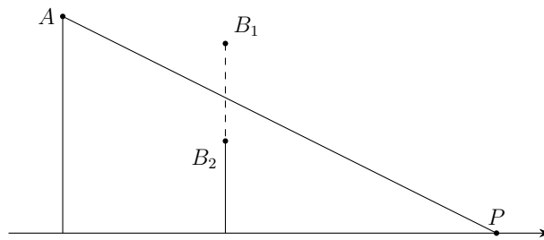
Figura 27.1: Privind din punctul P , stîlpul B_1 maschează stîlpul A complet, dar stîlpul B_2 nu. De aceea, vrăjitorul P l-ar prefera pe B_1 față de A ca mentor, dar l-ar prefera pe A față de B_2 .
