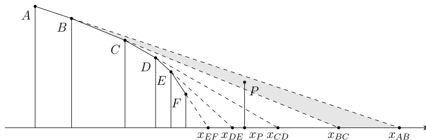
Figura 27.2: Mentorul vrăjitorului P este D deoarece x_P se află în triunghiul lui D . Mai mult, punctul P se află în triunghiul lui B , deci vrăjitorii C - F nu vor mai fi mentori niciodată.
