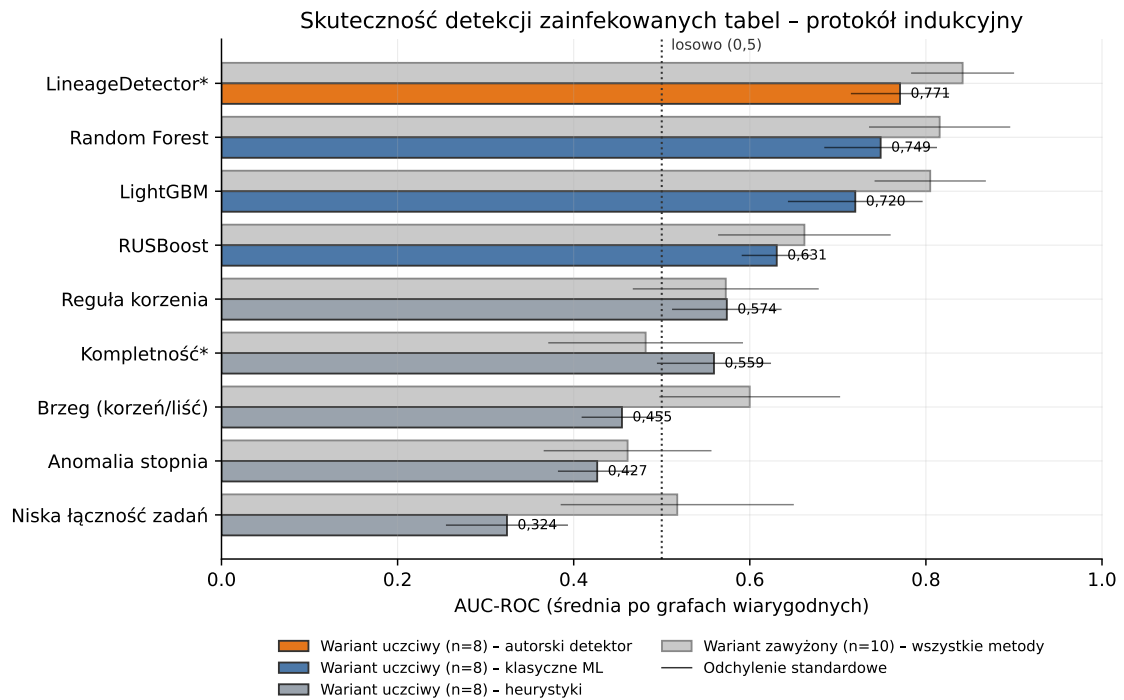
RYSUNEK 4.1: Porównanie AUC-ROC metod detekcji w wariancie ucziwym (z wykluczeniem węzłów izolowanych) i zawyzonym. Dla każdej metody dolny, kolorowy słupek przedstawia wariant ucziwy, a górny, jasnoszary słupek wariant zawyzony. Kolor słupka wariantu ucziwego oznacza grupę metod (pomarańczowy – autorski detektor, niebieski – klasyczne metody uczenia maszynowego, szary – heurystyki strukturalne). Poziome odcinki na końcach słupków pokazują odchylenie standardowe po grafach wiarygodnych, a pionowa linia kropkowana poziom losowy (AUC-ROC = 0,5). Gwiazdką oznaczono wkład własny. Metody uczone zachowują przewagę obu wariantach, a heurystyki lokalne tracą najwięcej po usunięciu przecieku izolacji.
