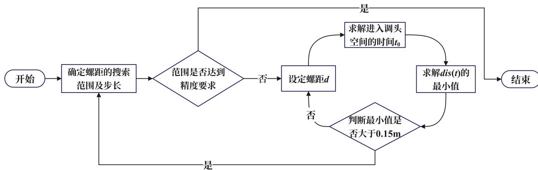
图 10 问题三求解流程图
