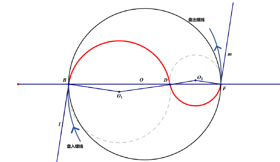
图 16 调头曲线示意图
