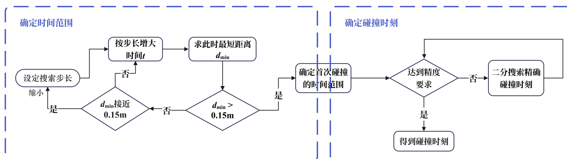
图 7 问题二求解流程图
