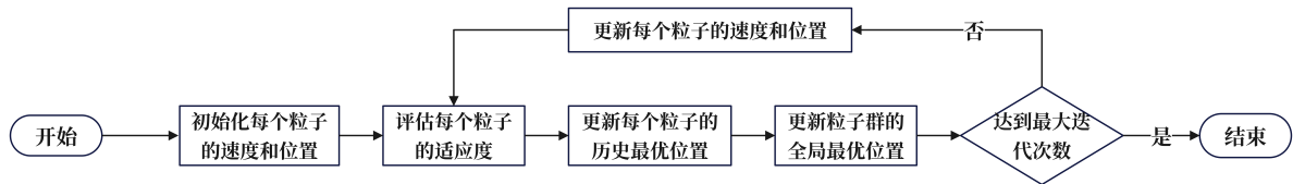
图 11 粒子群 (PSO) 算法流程图
