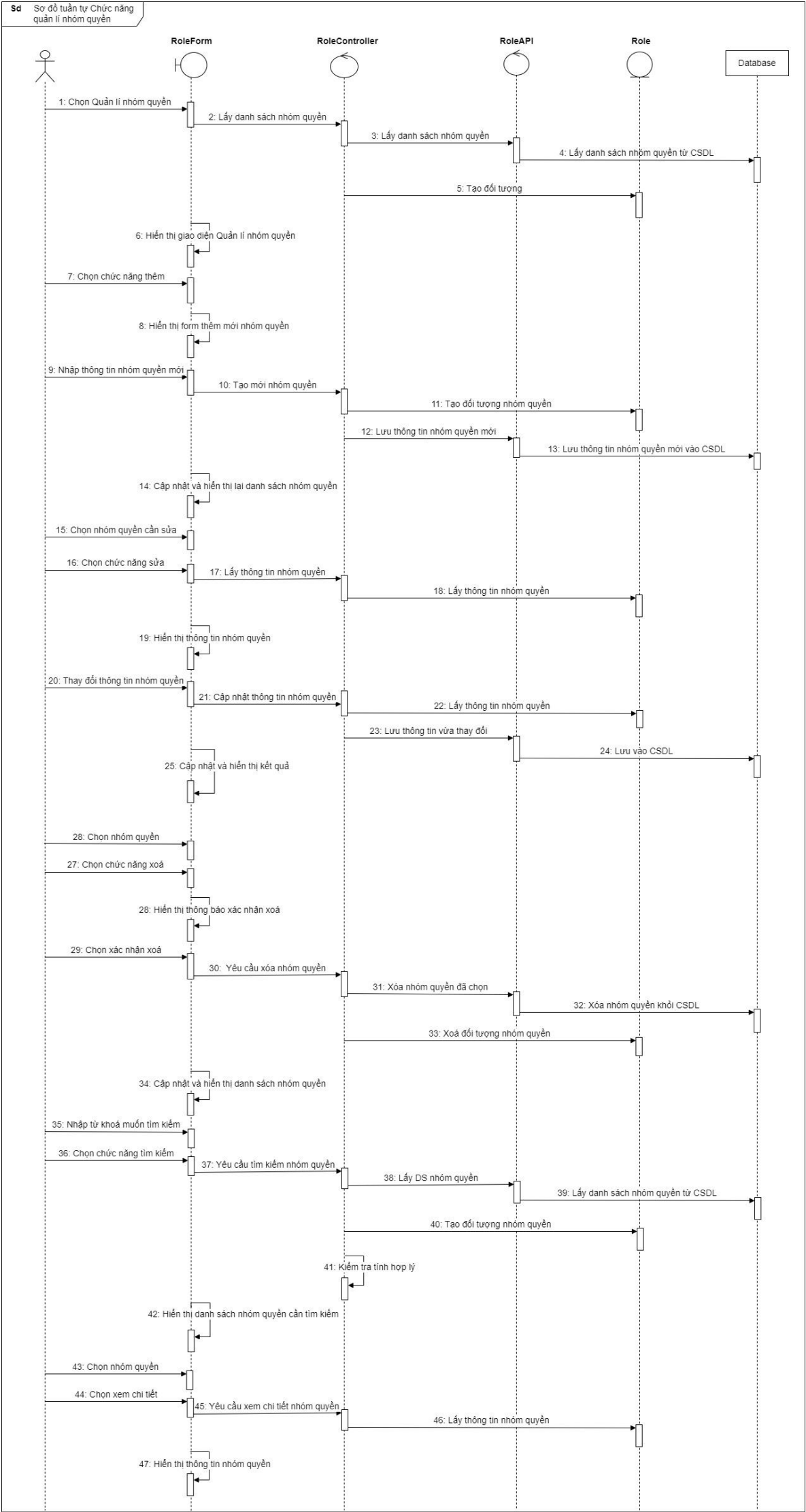
Hình 2.11 Biểu đồ tuần tự chức năng Quản lí nhóm quyền
