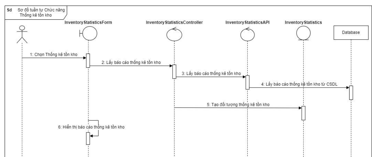
Hình 2.31 Biểu đồ tuần tự chức năng Thống kê tồn kho
