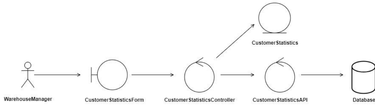
Hình 2.32 Sơ đồ lớp phân tích chức năng Thống kê khách hàng
