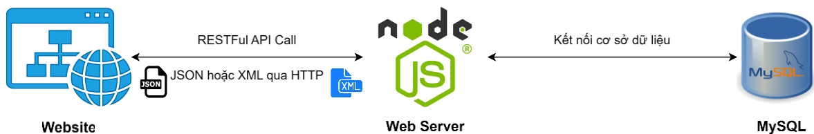
Hình 4.1 Sơ đồ triển khai hệ thống
