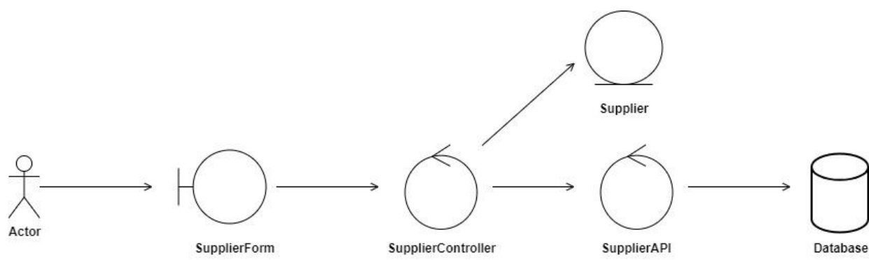
Hình 2.22 Sơ đồ lớp phân tích chức năng Quản lí nhà cung cấp
