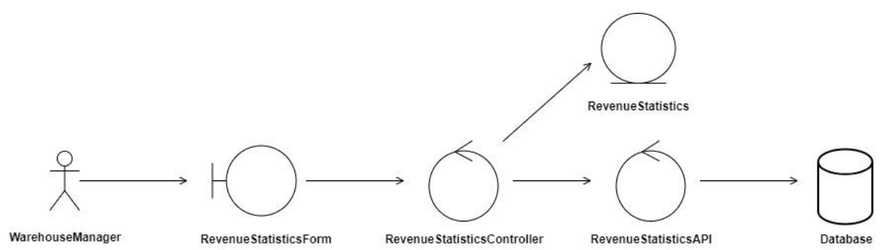
Hình 2.28 Sơ đồ lớp phân tích chức năng Thống kê doanh thu
