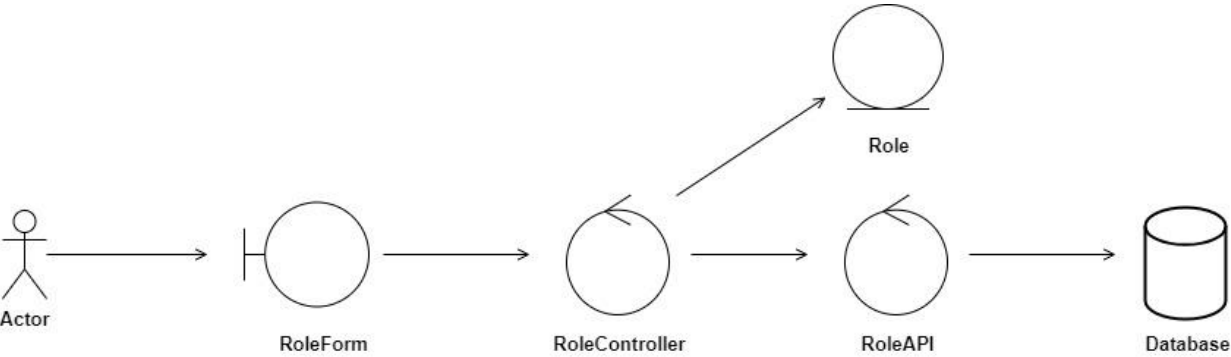
Hình 2.10 Sơ đồ lớp phân tích chức năng Quản lí nhóm quyền
