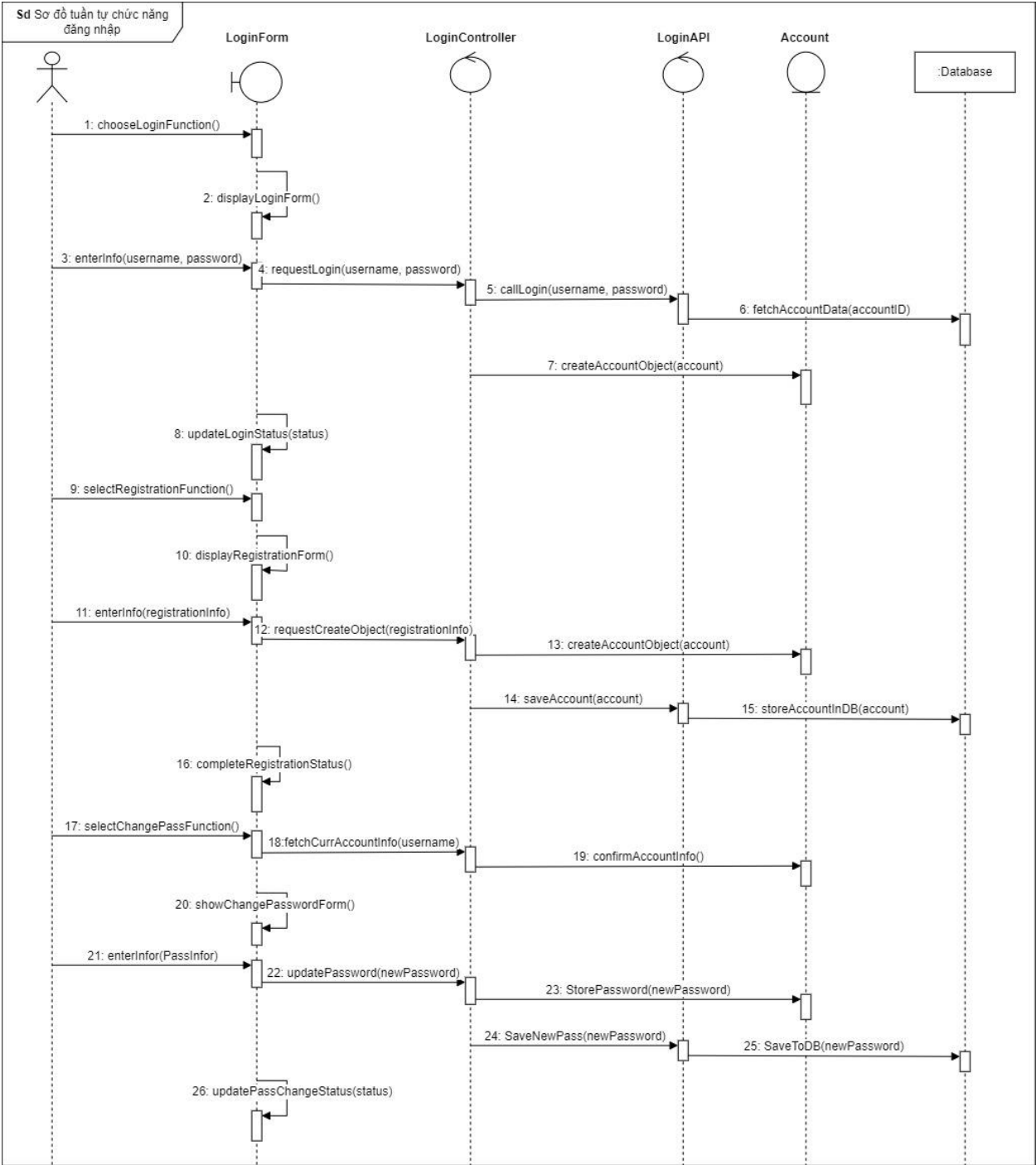
Hình 3.1 Biểu đồ tuần tự chức năng đăng nhập
