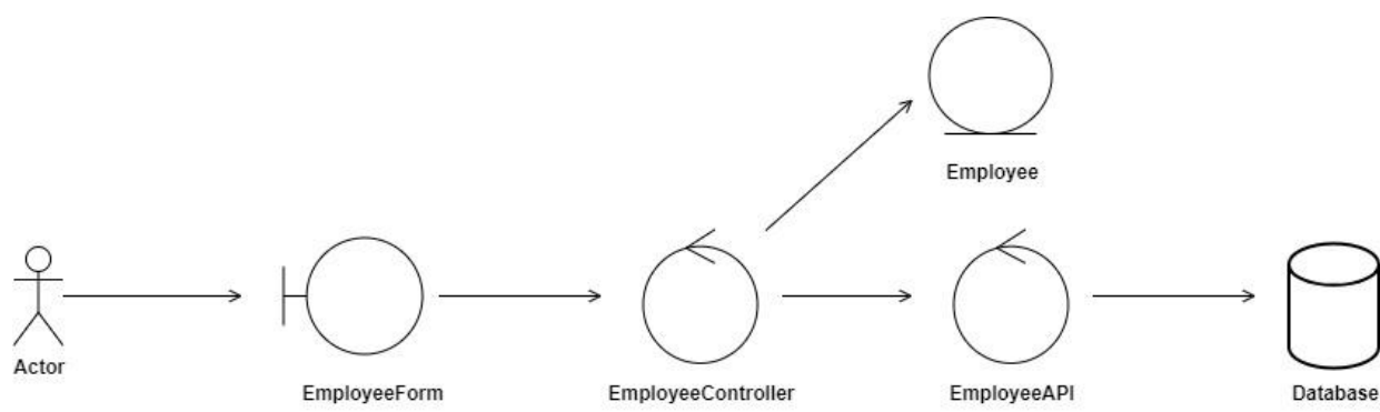
Hình 2.8 Sơ đồ lớp phân tích của chức năng Quản lí nhân viên
