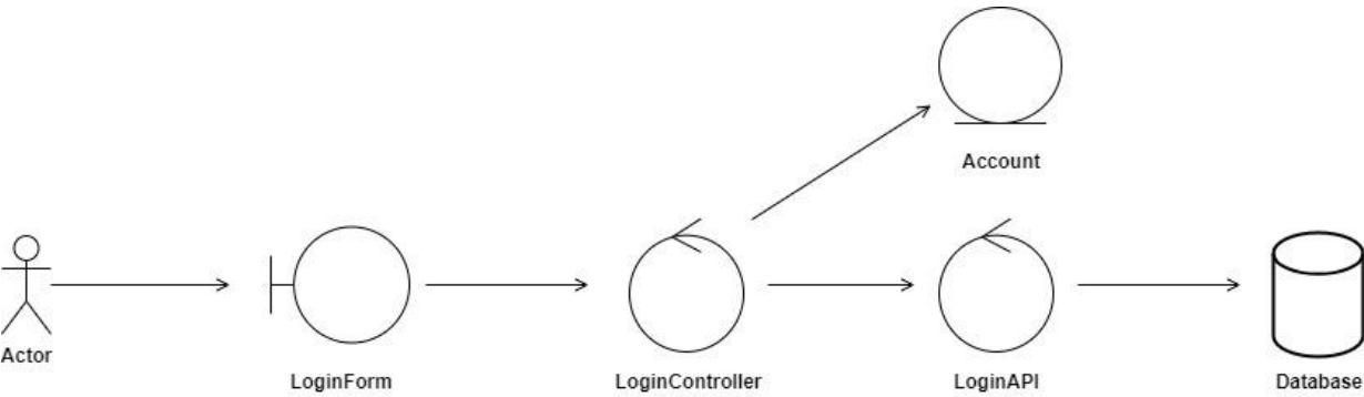
Hình 2.4 Sơ đồ lớp phân tích của chức năng Đăng nhập
