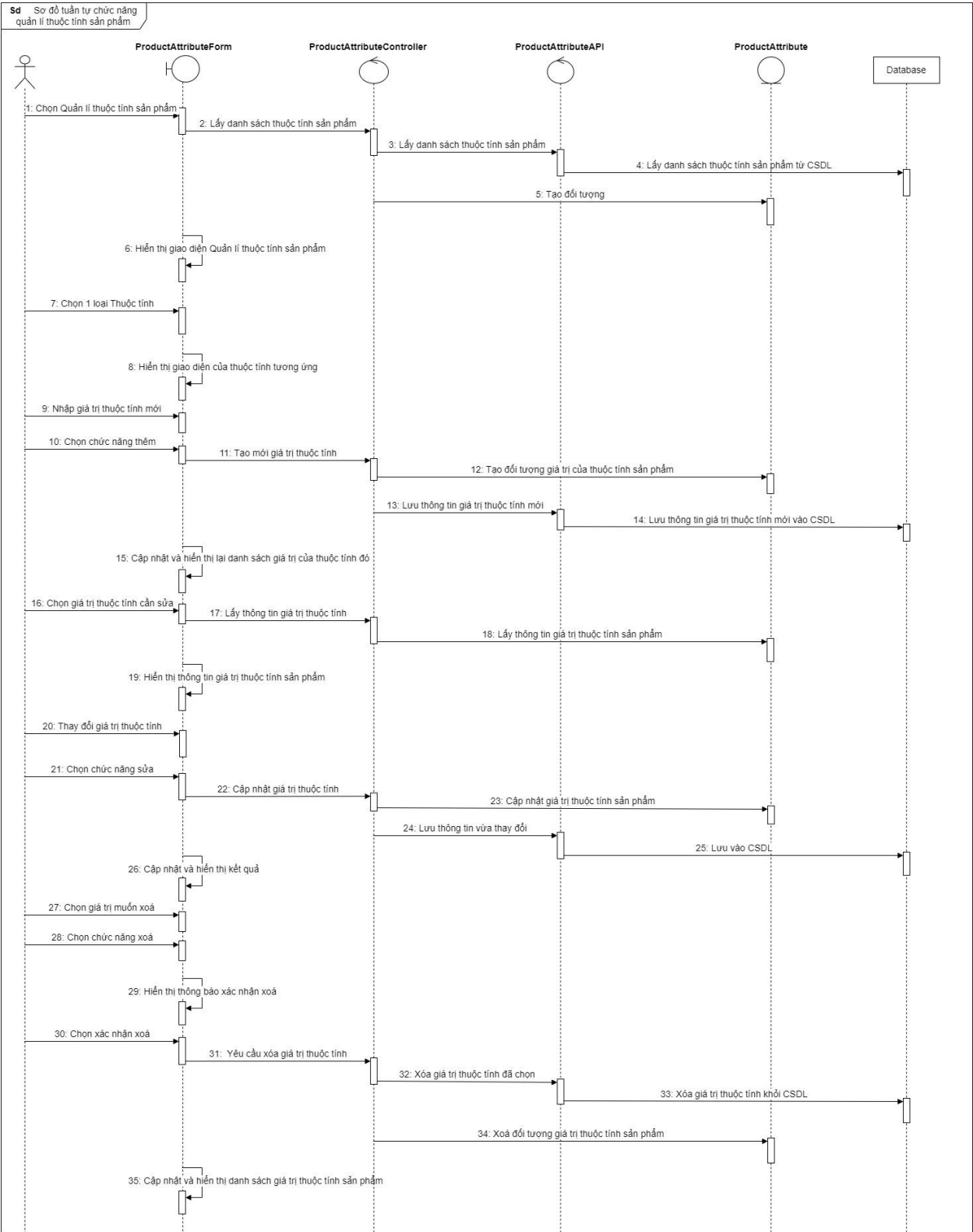
Hình 2.15 Biểu đồ tuần tự chức năng Quản lý thuộc tính sản phẩm
