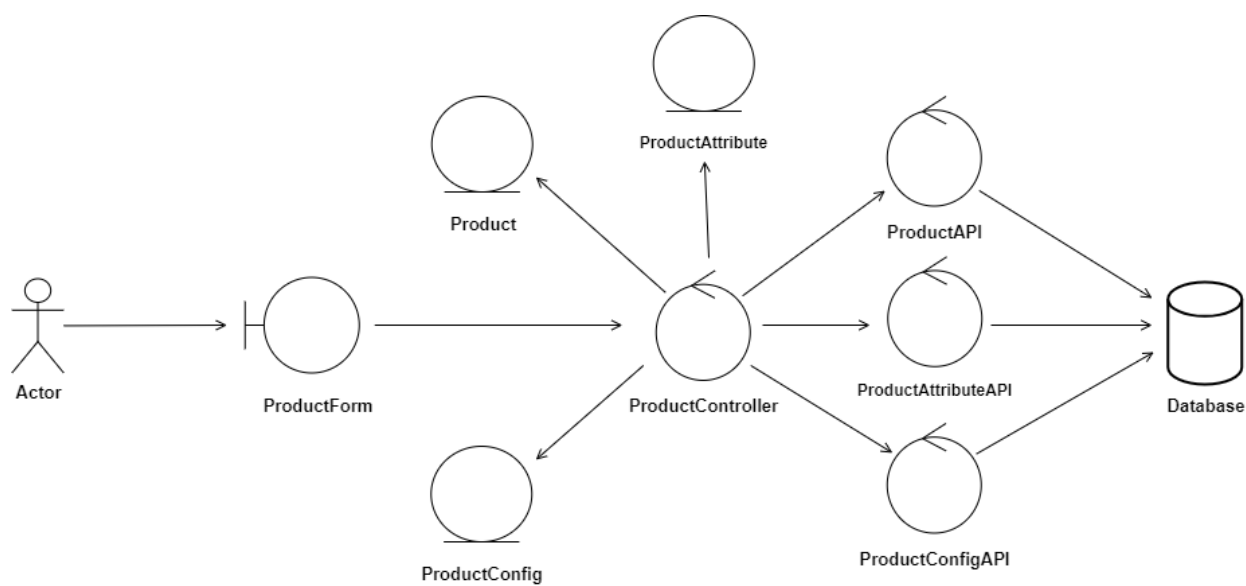
Hình 2.12 Sơ đồ lớp phân tích chức năng Quản lí sản phẩm
