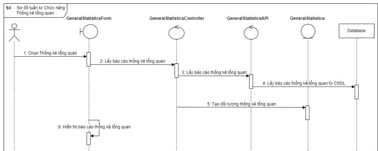
Hình 2.27 Biểu đồ tuần tự chức năng Thống kê tổng quan
