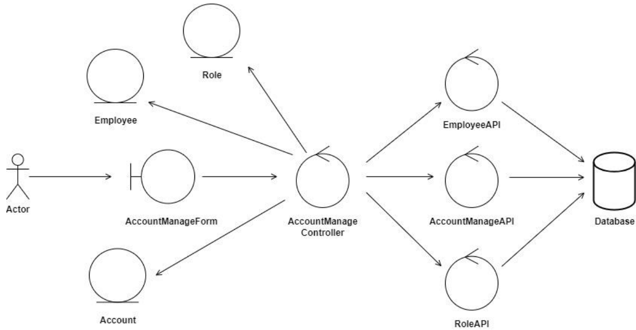
Hình 2.6 Sơ đồ lớp phân tích của chức năng Quản lí tài khoản người dùng
