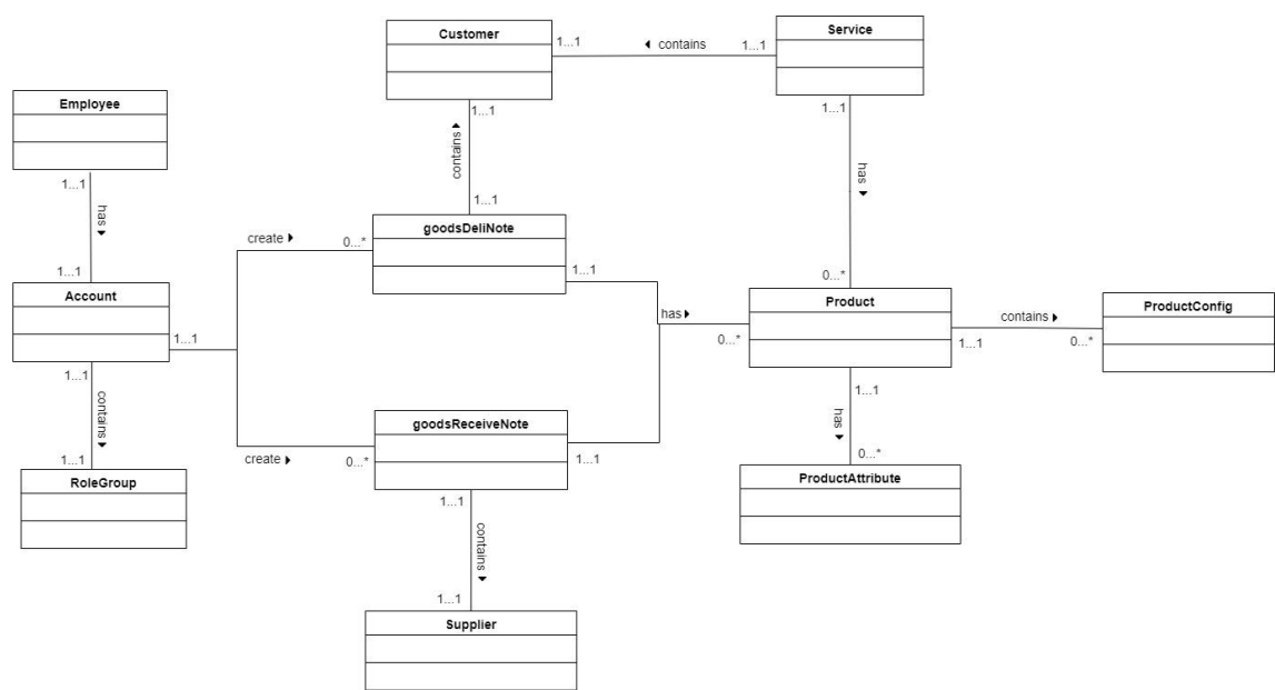
Hình 3.11 Biểu đồ lớp
