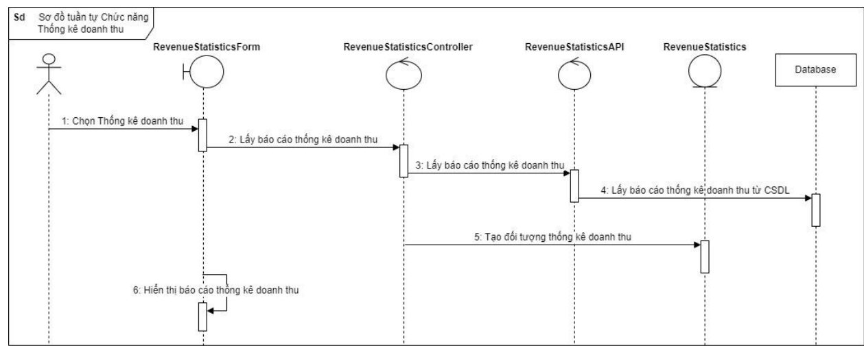
Hình 2.29 Biểu đồ tuần tự chức năng Thống kê doanh thu
