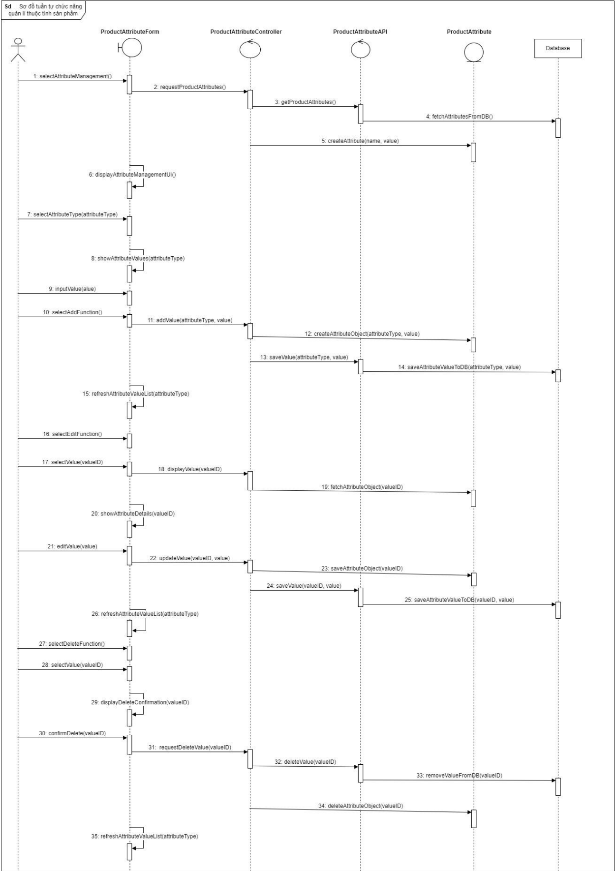
Hình 3.6 Biểu đồ tuần tự chức năng quản lý thuộc tính sản phẩm
