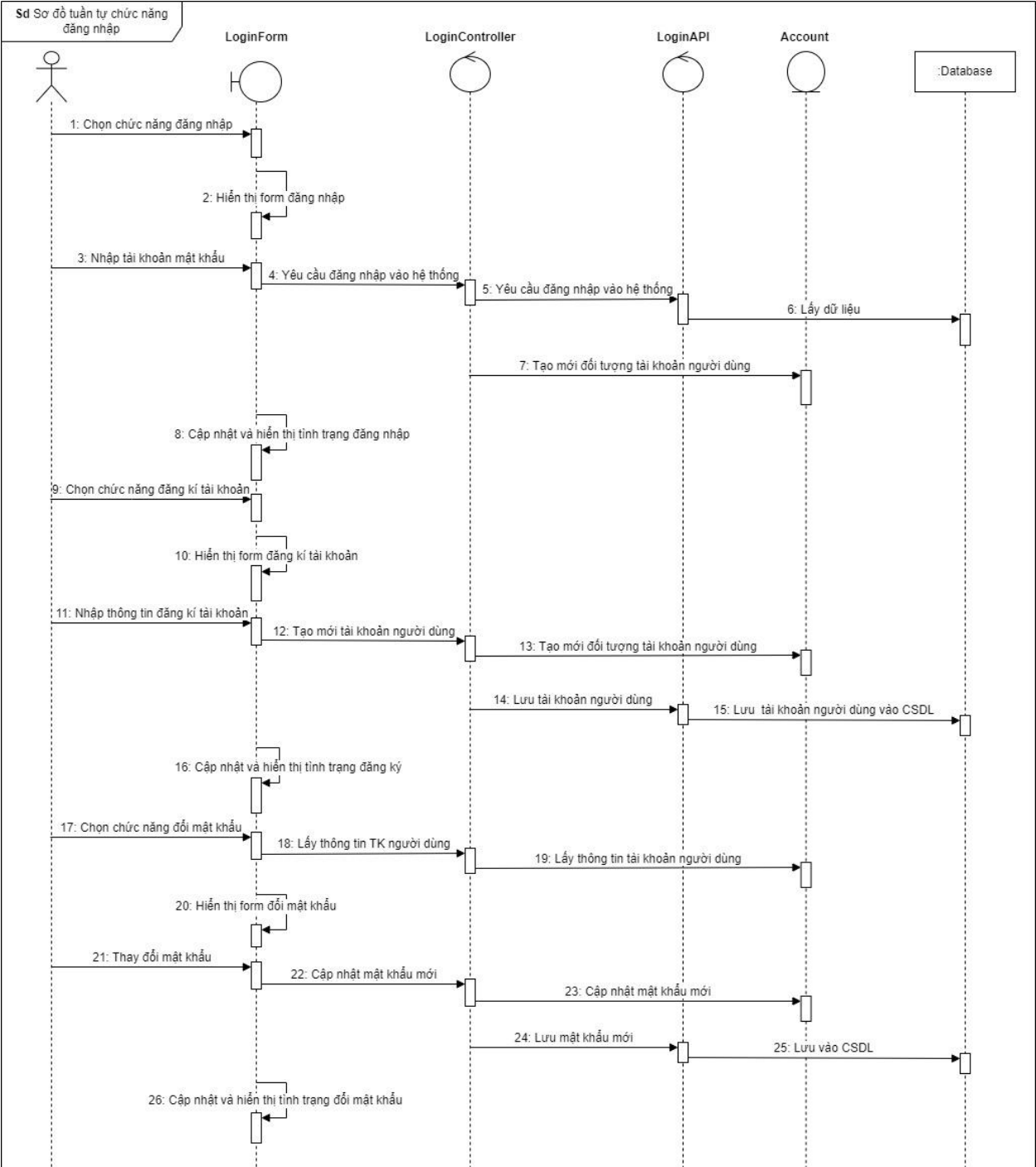
Hình 2.5 Sơ đồ tuần tự của chức năng Đăng nhập
