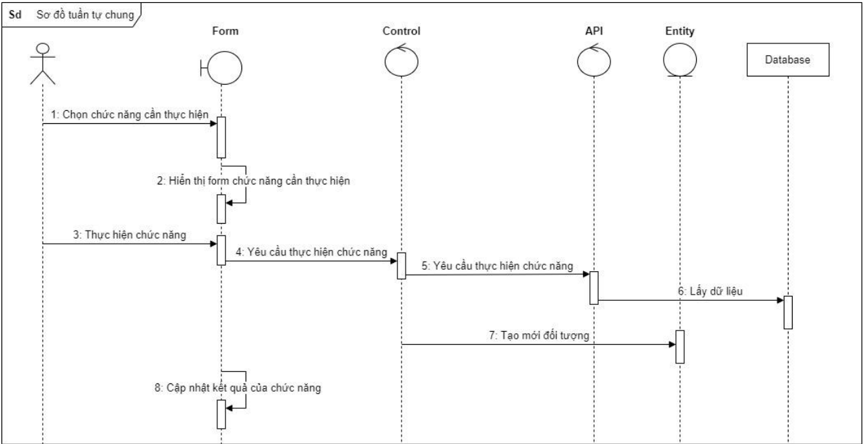
Hình 2.3 Sơ đồ tuần tự chung
