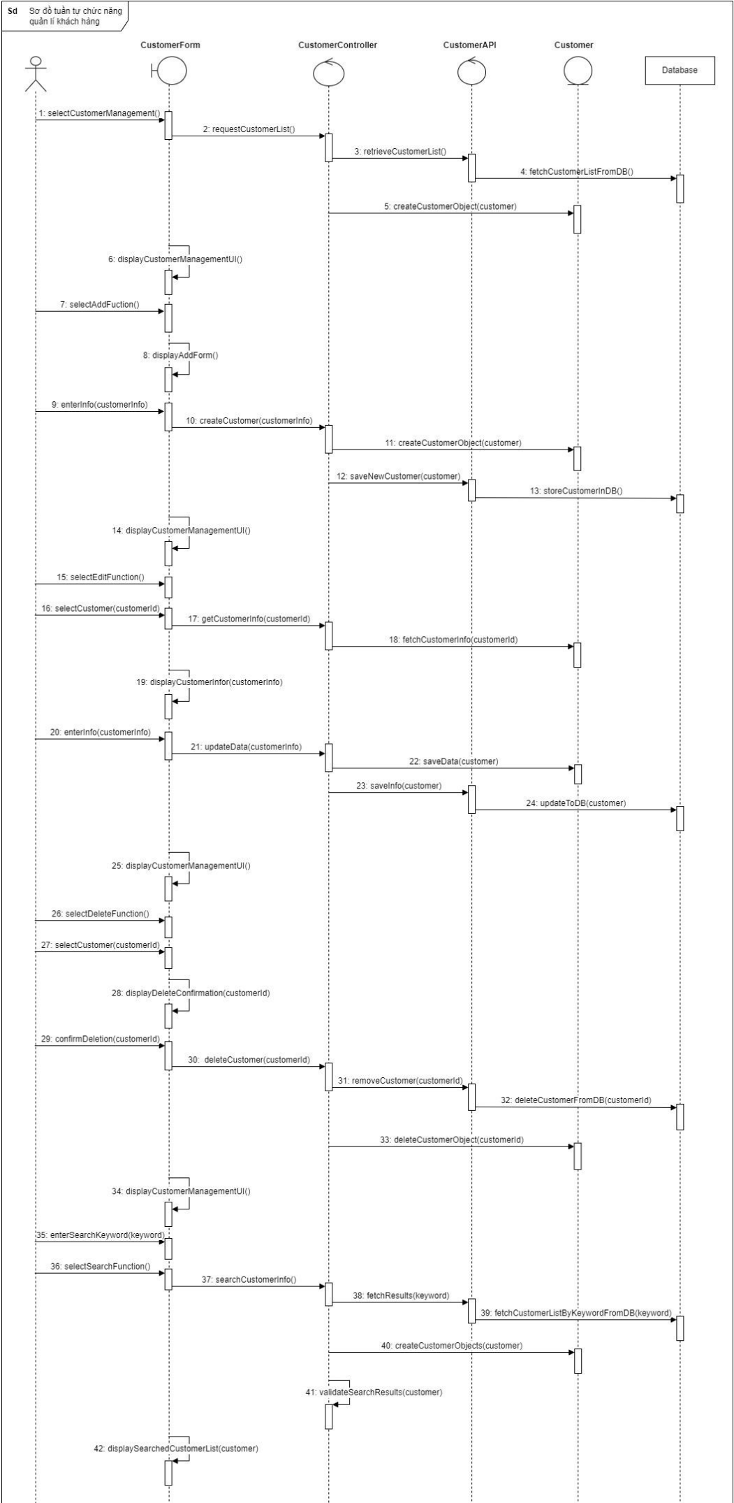
Hình 3.7 Biểu đồ tuần tự chức năng quản lí khách hàng
