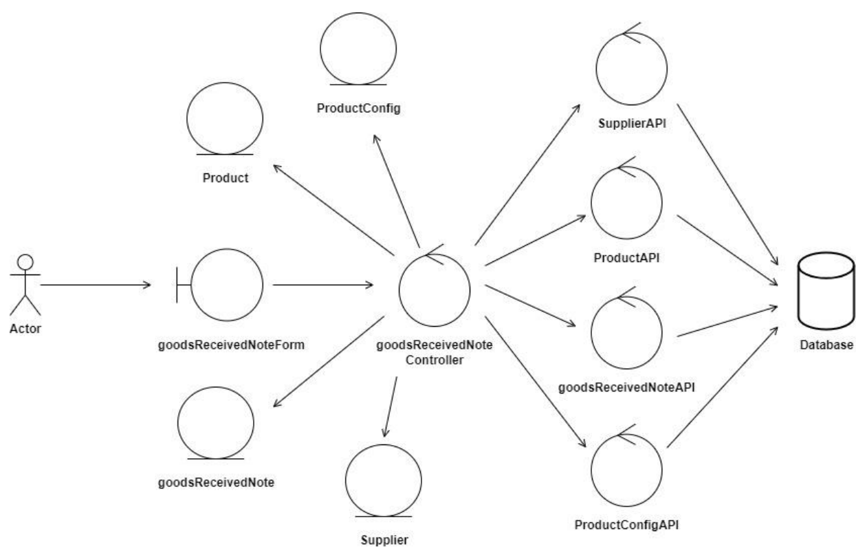
Hình 2.16 Sơ đồ lớp phân tích chức năng Quản lí nhập kho
