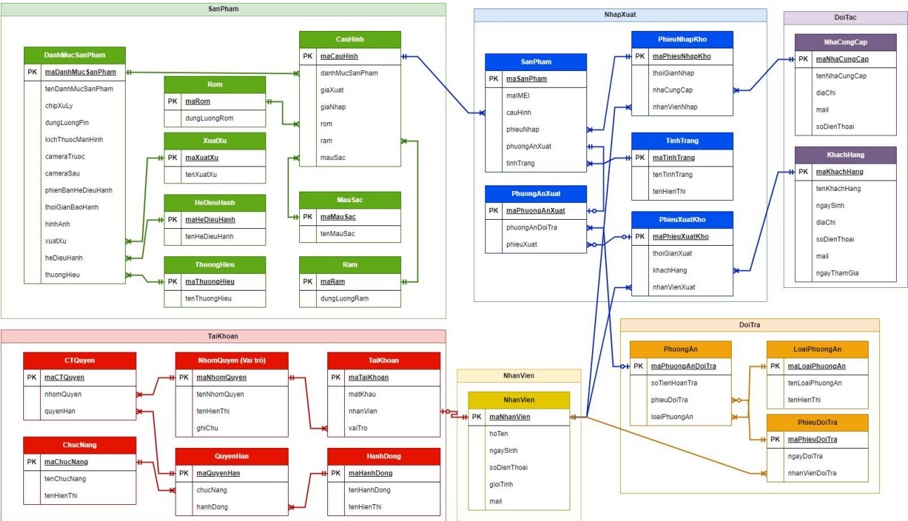
Hình 3.12 Lược đồ cơ sở dữ liệu
