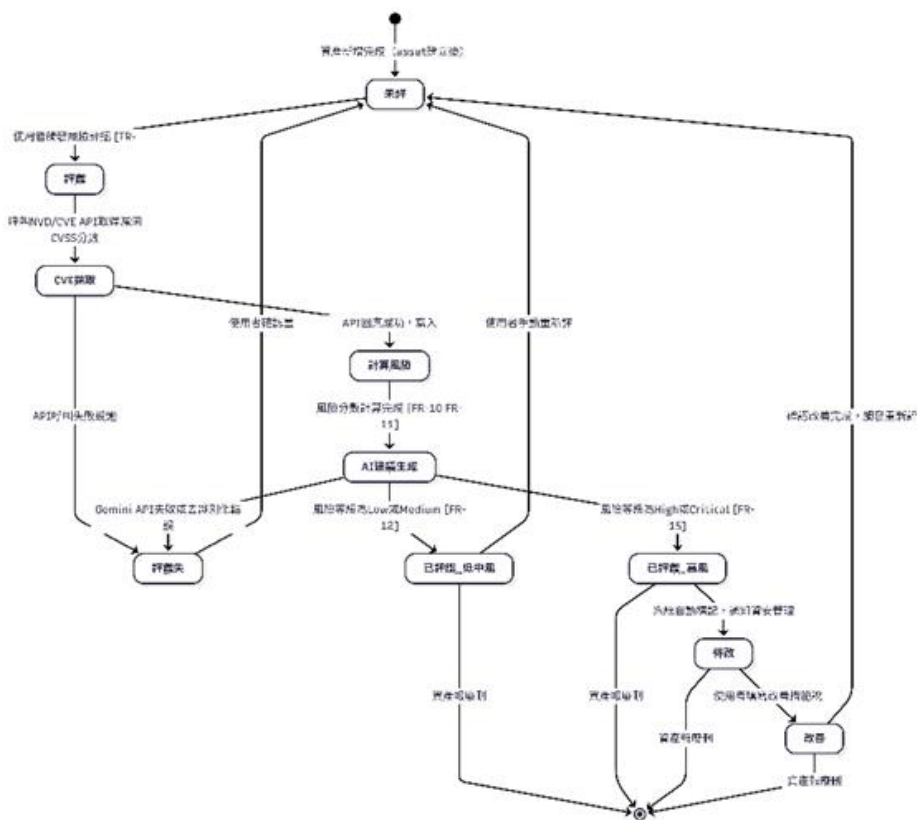
圖 7-4-1 狀態機圖
