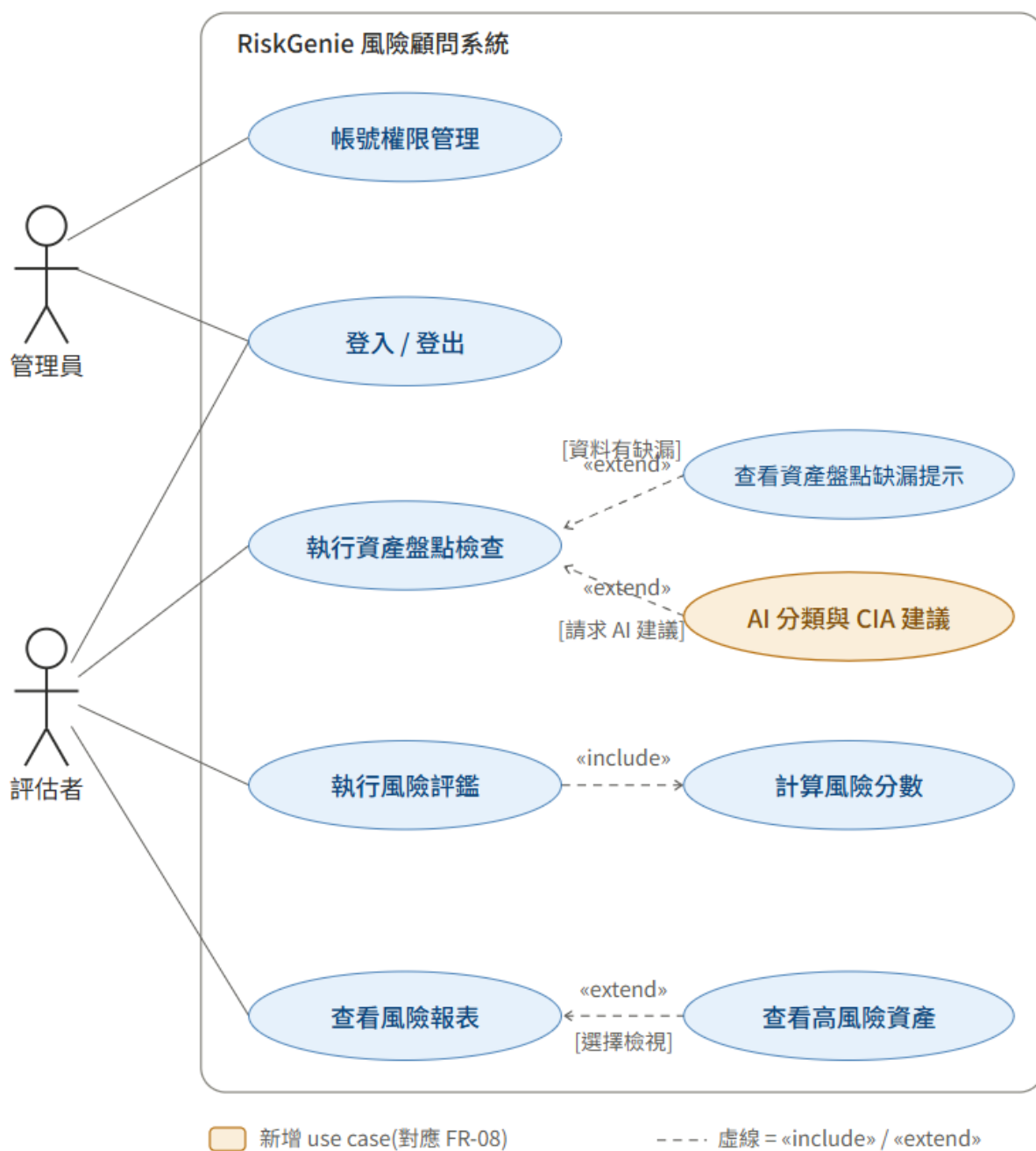
圖 5-2-1 使用個案圖
