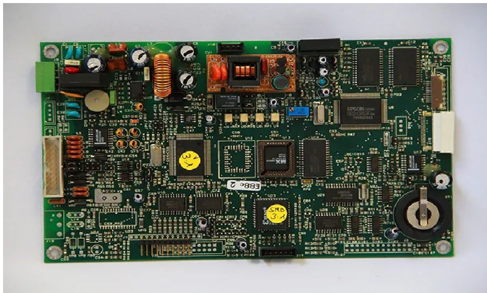
Imagem da placa mostrando os pontos de teste marcados
