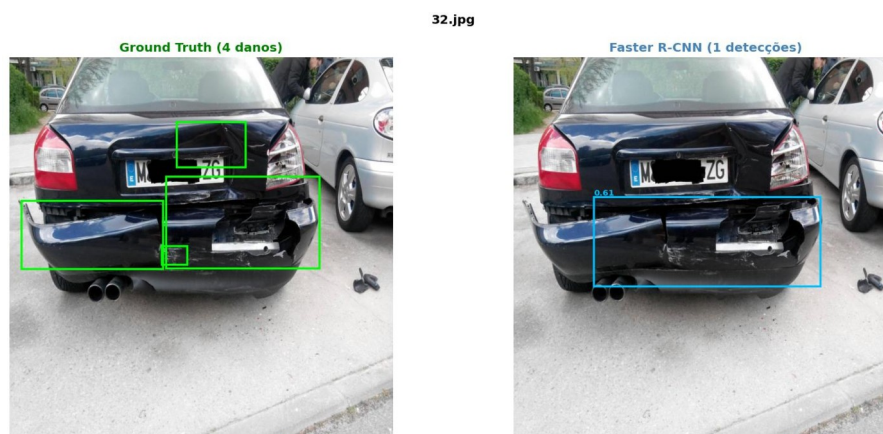
Figura 3 – Resultado da avaliação do Faster R-CNN na primeira rodada de treinamento Fonte: Elaborada pelo autor (2026).
