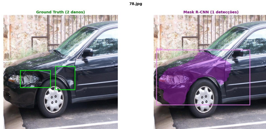
Figura 4 – Resultado da avaliação do Mask R-CNN na primeira rodada de treinamento
