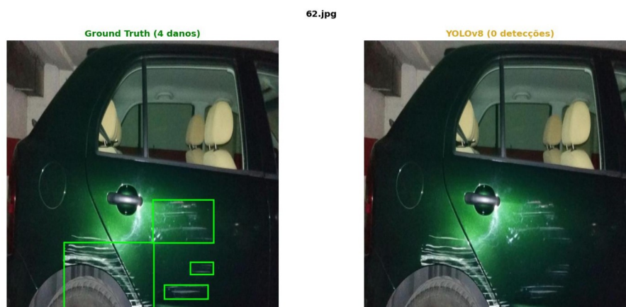
Figura 2 – Resultado da avaliação do YOLOv8 na primeira rodada de treinamento Fonte: Elaborada pelo autor (2026).
