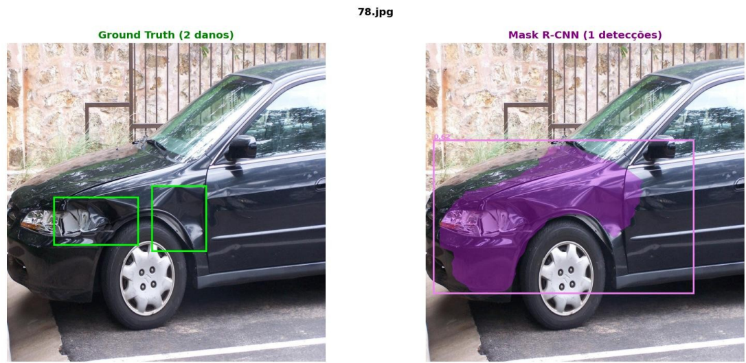
Figura 4 – Resultado da avaliação do Mask R-CNN na primeira rodada de treinamento Fonte: Elaborada pelo autor (2026).
