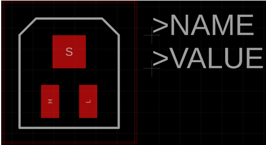
Obudowa 1814
