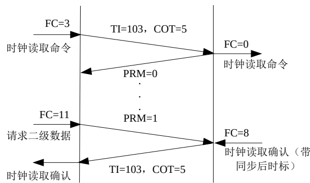
图 7 非平衡链路传输模式中时钟读取过程
