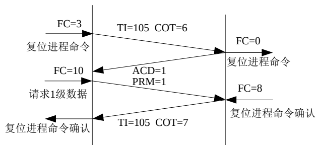
图 19 非平衡链路模式下的复位进程过程
