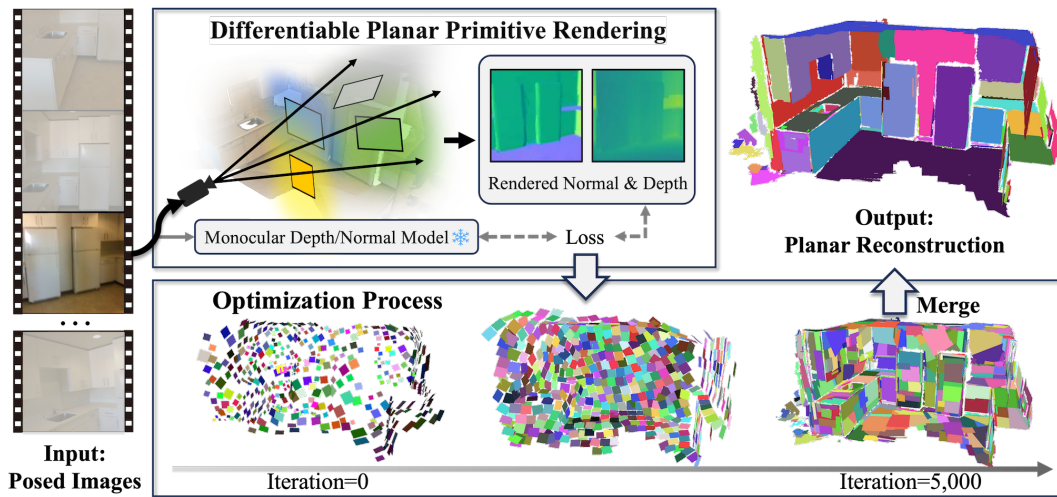
FIGURA 2.1: Arquitectura general de PlanarSplatting. El método optimiza primitivas planas 3D directamente desde imágenes multi- vista empleando renderizado diferenciable. Esto permite evadir la densificación clásica de MVS y obtener modelos ultrarrápidos (Fuente: [11]).
