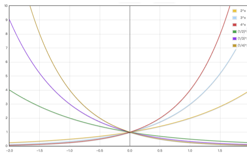
图 2: 指数函数的图象
