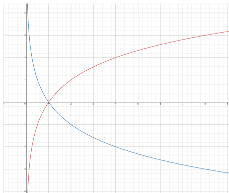
图 4: 对数函数的图象
