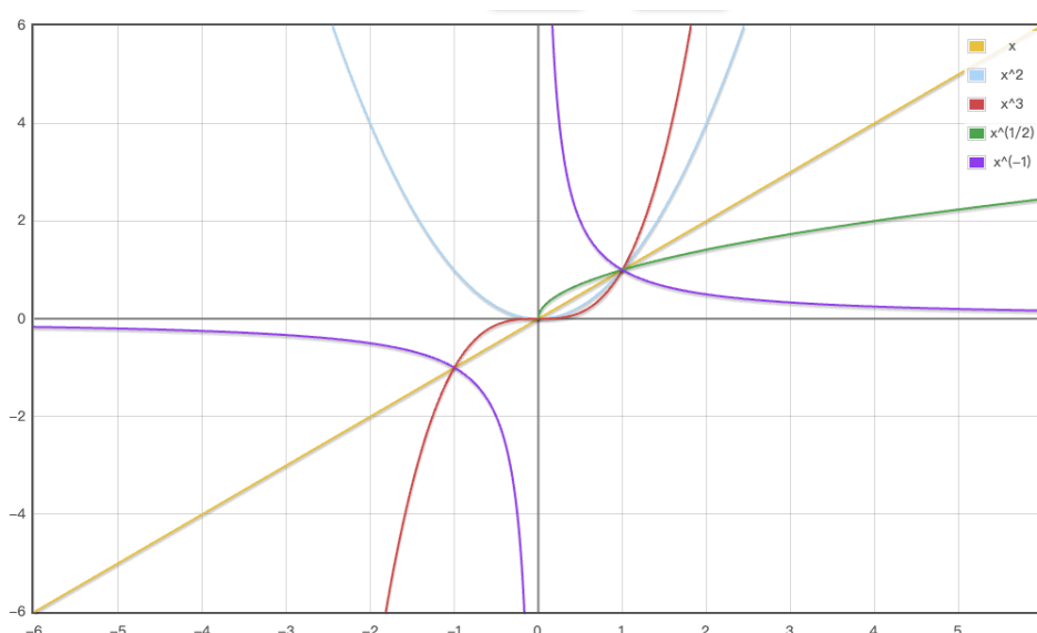
图 1: 幂函数的图象
