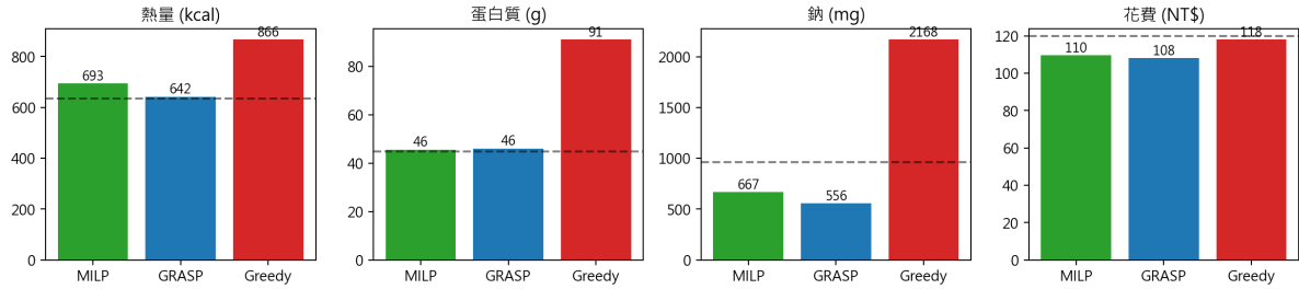
Figure 1: U1 男·減脂·正餐情境 (488 項真實全家商品) 下三種解法之熱量、蛋白質、鈉與成本對比 (虛線為對應限制)。MILP 解為結構完整的一餐：小菠蘿麵包 (主餐) + 蜜汁豬肉乾 (配菜) + 無加糖濃豆漿 (飲料) + 綜合水果軟糖 (甜點)，總價 NT$110、693 kcal、45.6 g 蛋白質、667 mg 鈉，全部達標；GRASP-LS 取另一近似最優之結構餐 (NT$108)。Greedy 為榨取「蛋白質／價格比」挑出雞腿排 + 豬耳絲 + 豆漿，缺主餐 (違反 C11)、鈉量 2168 mg 突破 1.5\times 硬上限 (違反 C8b)， hard-infeasible 。
