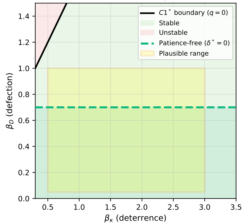
(1) Parameter Space
