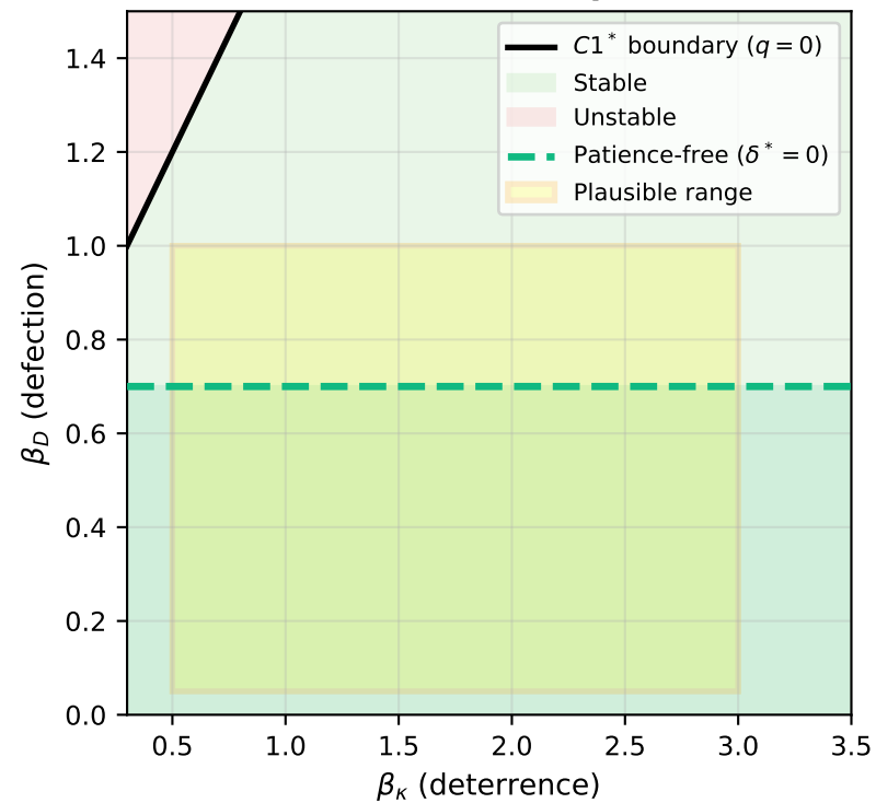
(1) Parameter Space
