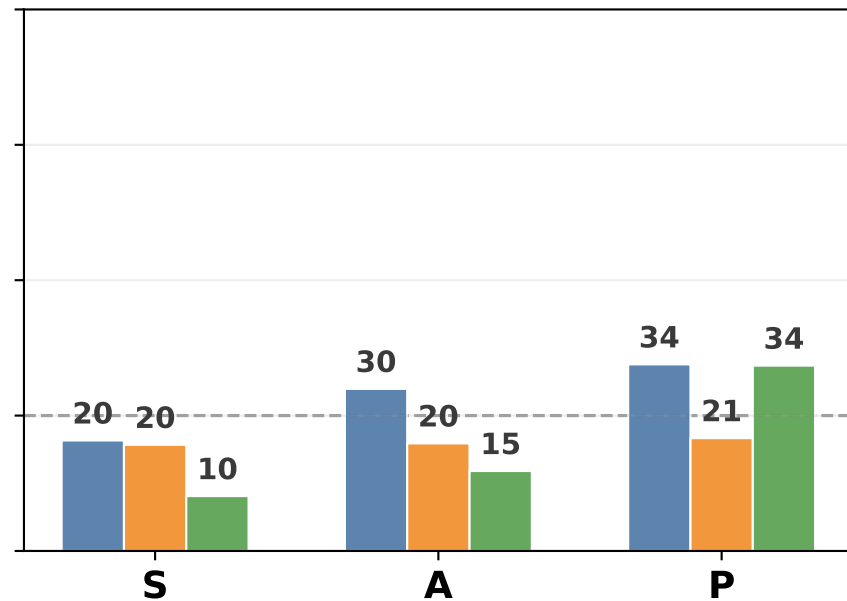
Qwen3-VL-8B
