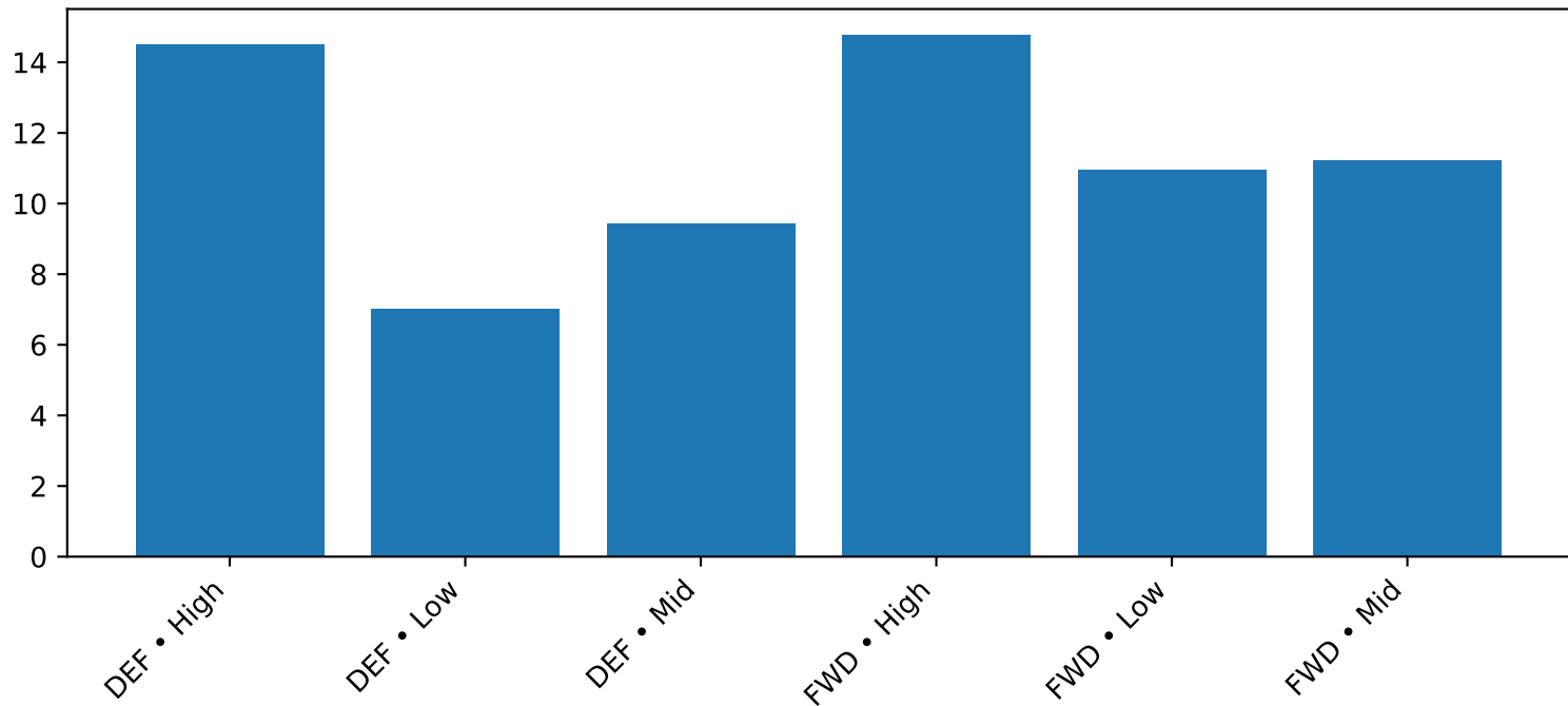
VAL — MAE par segment (macroxtier)
