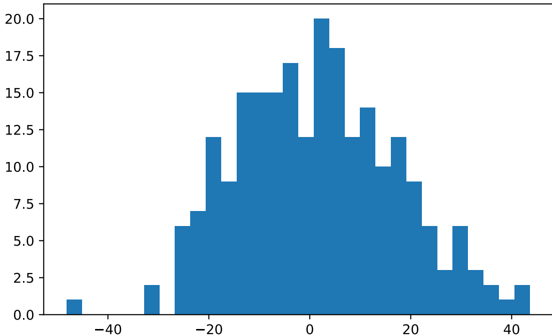
VAL — Histogramme des résidus ( y_{\text{true}} - y_{\text{pred}} )
