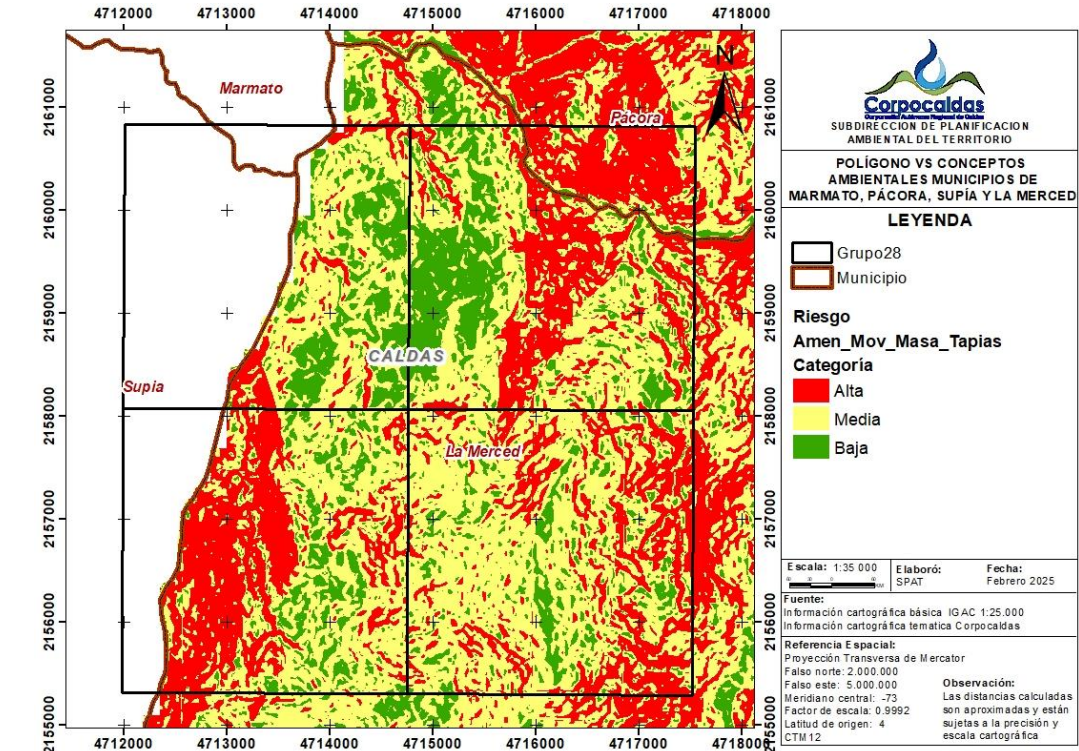
Figura 7. Áreas de amenaza por Movimiento en Masa que se superponen con el polígono solicitado. Fuente: Río Tapias y otros directos al Cauca
