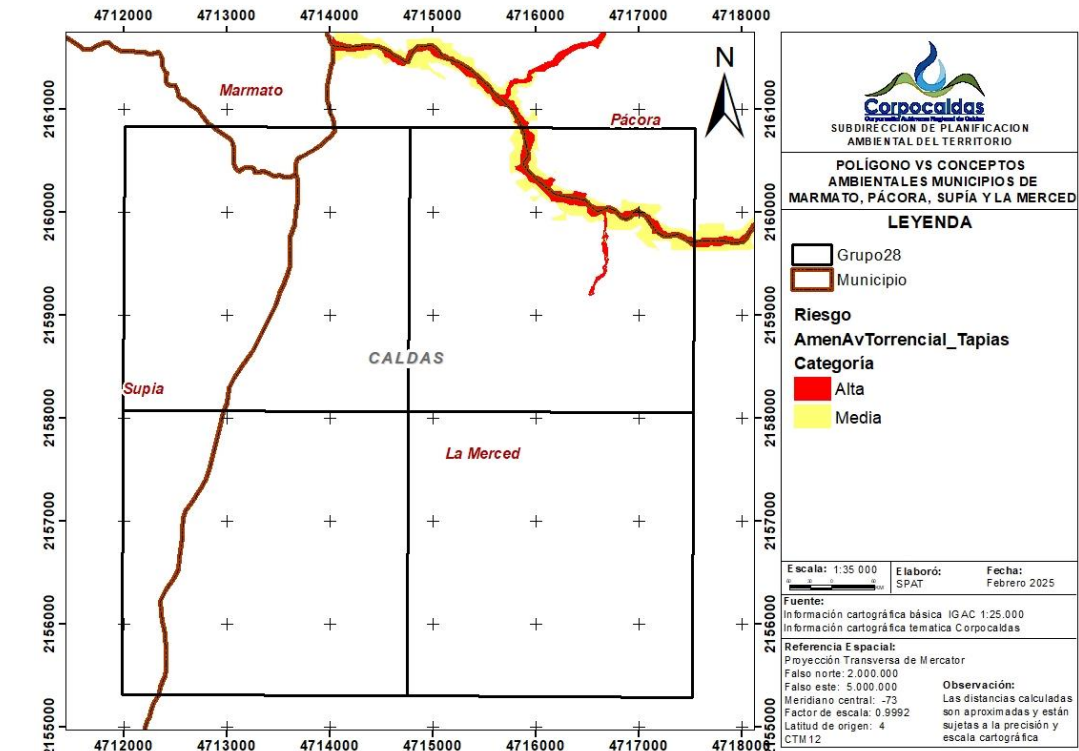
Figura 8. Áreas de amenaza por Avenida Torrencial que se superponen con el polígono solicitado. Fuente: Río Tapias y otros directos al Cauca
