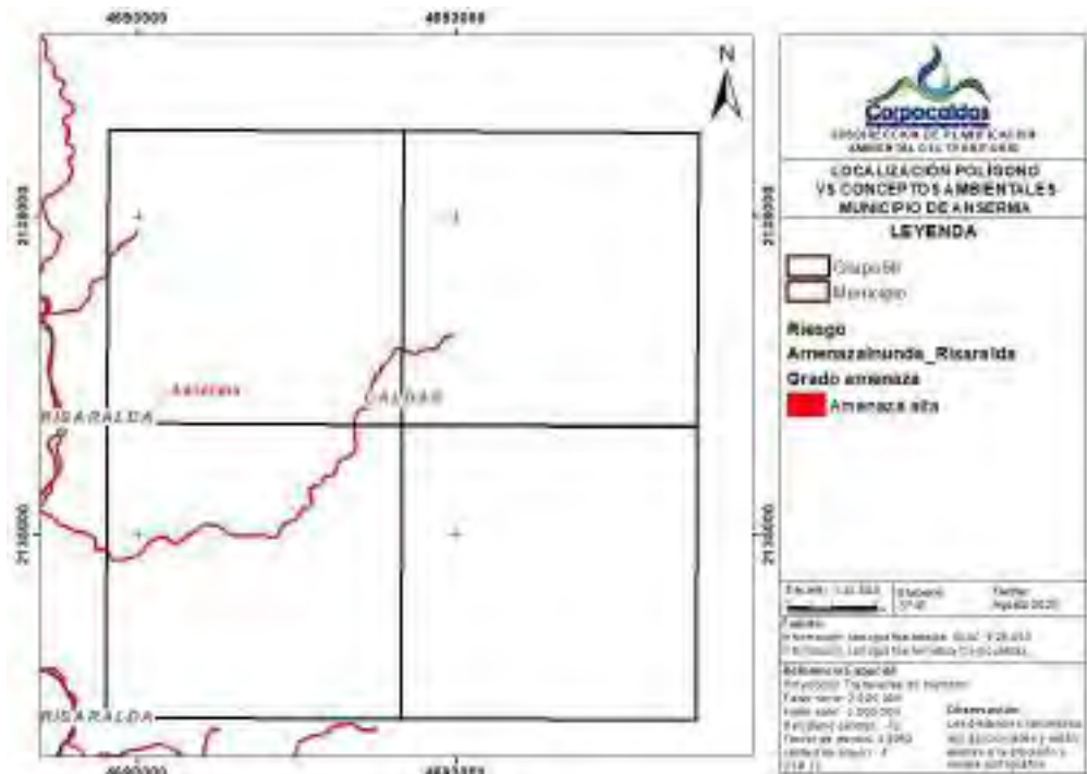
Figura 9. Áreas de amenaza por Inundación que se superponen con el polígono solicitado. Fuente: POMCA del río Risaralda
