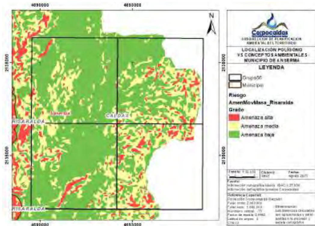
Figura 7. Áreas de amenaza por Movimiento en Masa que se superponen con el polígono solicitado. Fuente: POMCA del río Risaralda
