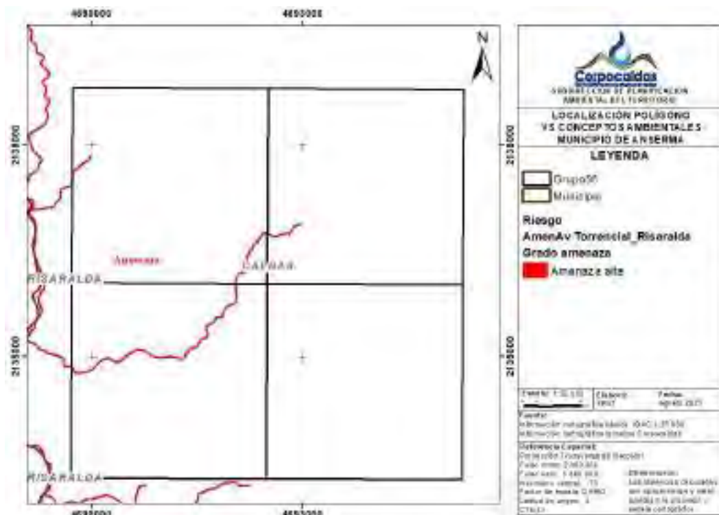
Figura 8. Áreas de amenaza por Avenida Torrencial que se superponen con el polígono solicitado. Fuente: POMCA del río Risaralda
