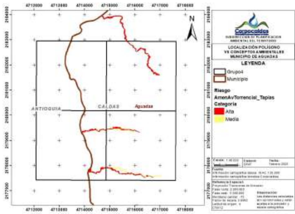
Figura 7. Áreas de amenaza por Avenida Torrencial que se superponen con el polígono solicitado. Fuente: POMCA río Tapias y otros directos al Cauca
