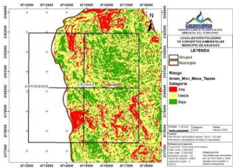
Figura 6. Áreas de amenaza por Movimiento en Masa que se superponen con el polígono solicitado. Fuente: POMCA río Tapias y otros directos al Cauca
