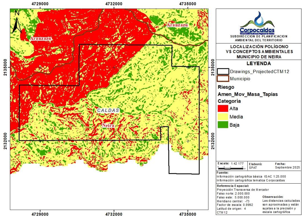
Figura 9. Áreas de amenaza por Movimiento en Masa que se superponen con el polígono solicitado. Fuente: POMCA del río Tapias y otros directos al Cauca
