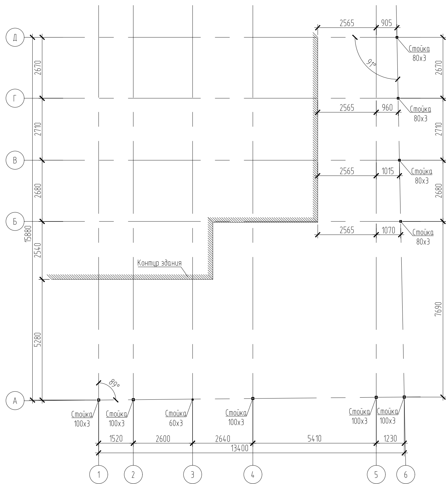
Схема расположения стоек
