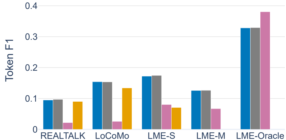
Token F1
