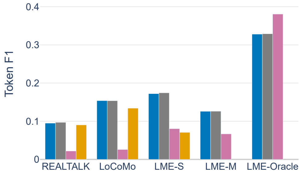
Token F1
