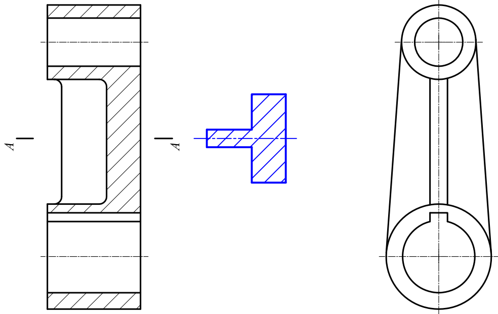
3. 画出指A-A断面图。
