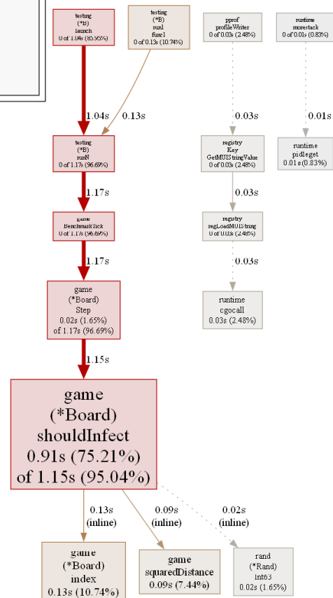
Figure — Graphe d'appels CPU (go tool pprof -png).
