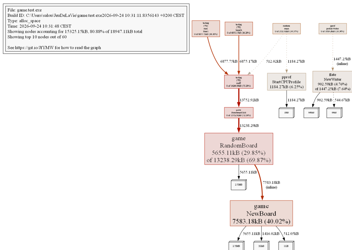
Figure — Graphe d'appels mémoire (go tool pprof -png).
