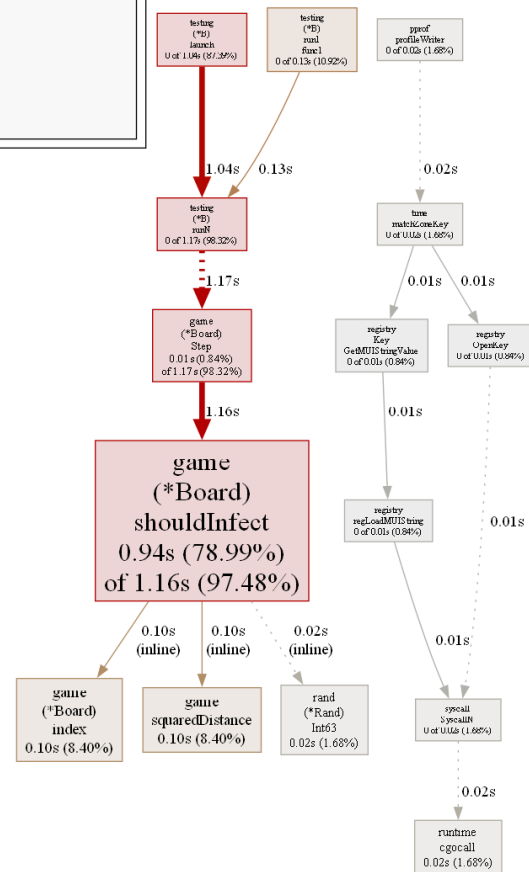
Figure — Graphe d'appels CPU (go tool pprof -png).
