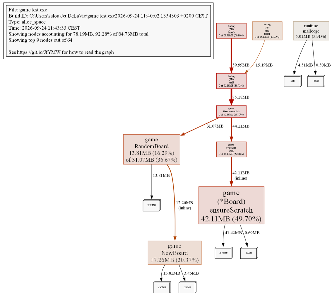
Figure — Graphe d'appels mémoire (go tool pprof -png).
