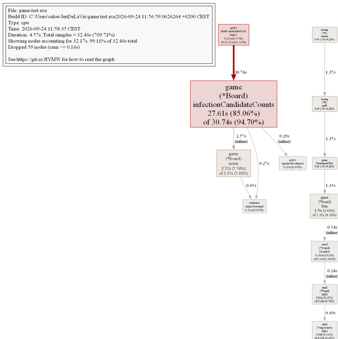
Figure — Graphe d'appels CPU (go tool pprof -png).
