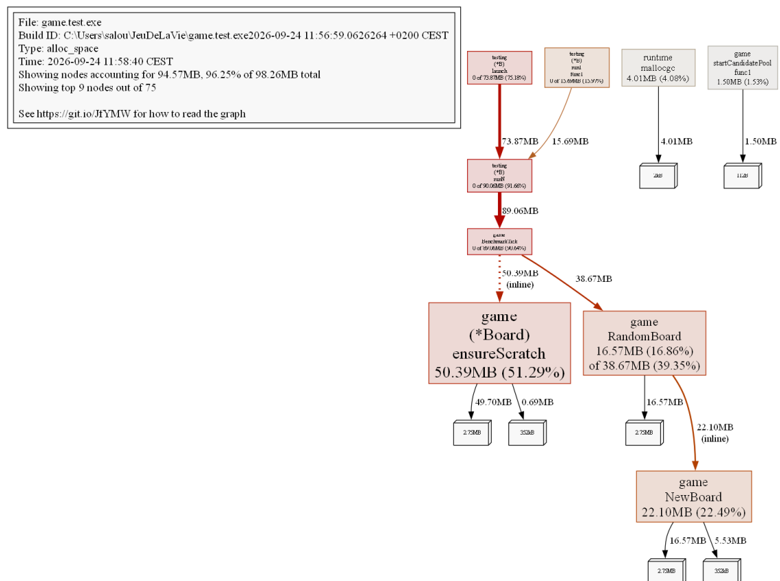
Figure — Graphe d'appels mémoire (go tool pprof -png).
