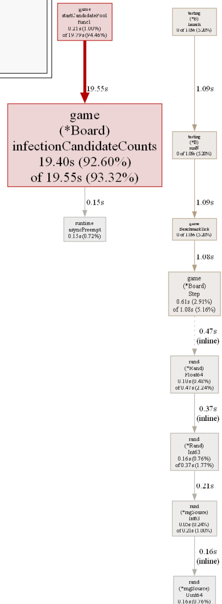
Figure — Graphe d'appels CPU (go tool pprof -png).
