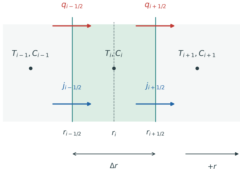
(b) 径向局部展开与共享通量
