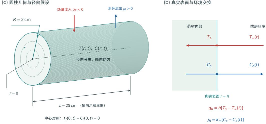
图 3: 问题一圆柱几何、径向坐标及真实表面 Robin 交换示意
