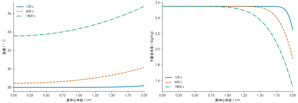
图 5: 预热阶段不同时刻的径向温度与含水率剖面
