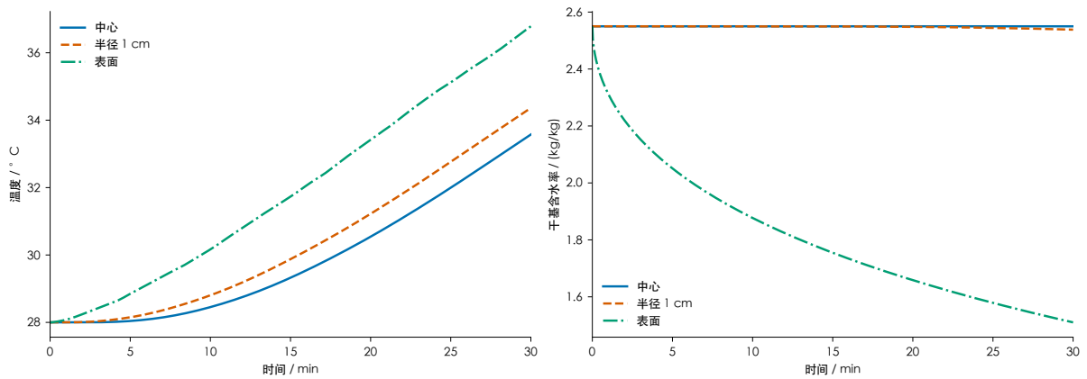
图 6: 中心、内部位置与表面的温度和含水率随时间的变化
