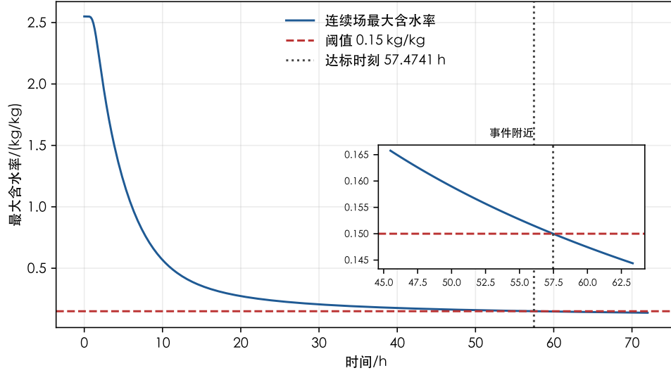
图 9: 问题三全域最大含水率与达标事件
