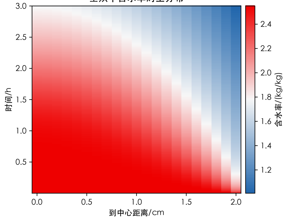
全烘干含水率时空分布
